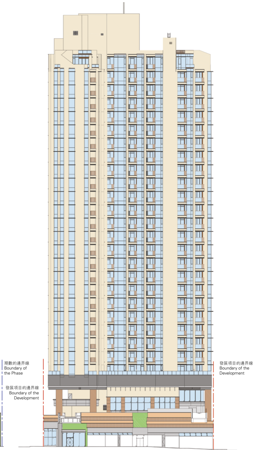
立面圖 4 ELEVATION PLAN 4
