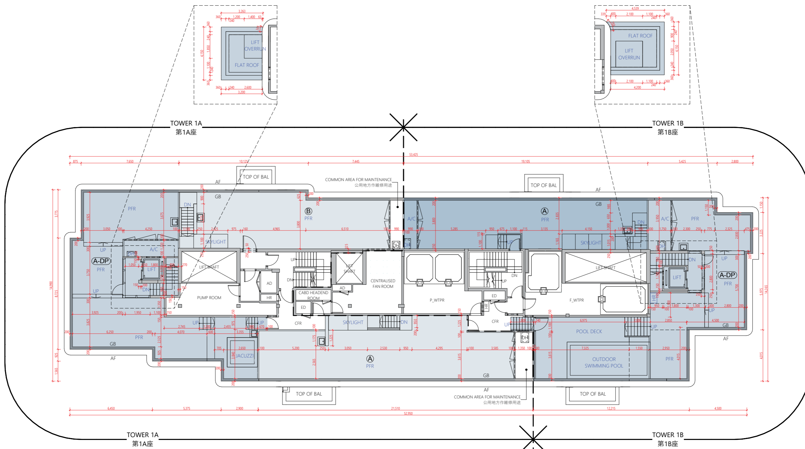
PART PLAN OF TOWER 1B FLAT A-DP UPPER ROOF 第1B座A-DP單位之上層天台部分平面圖
