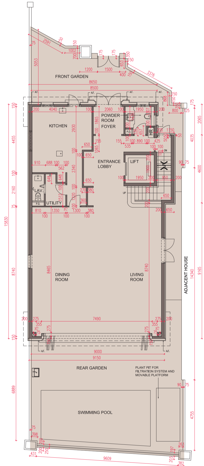
GROUND FLOOR PLAN 地下平面圖
