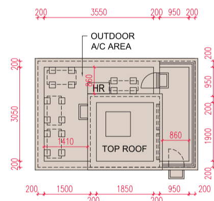
TOP ROOF FLOOR PLAN 上層天台平面圖
