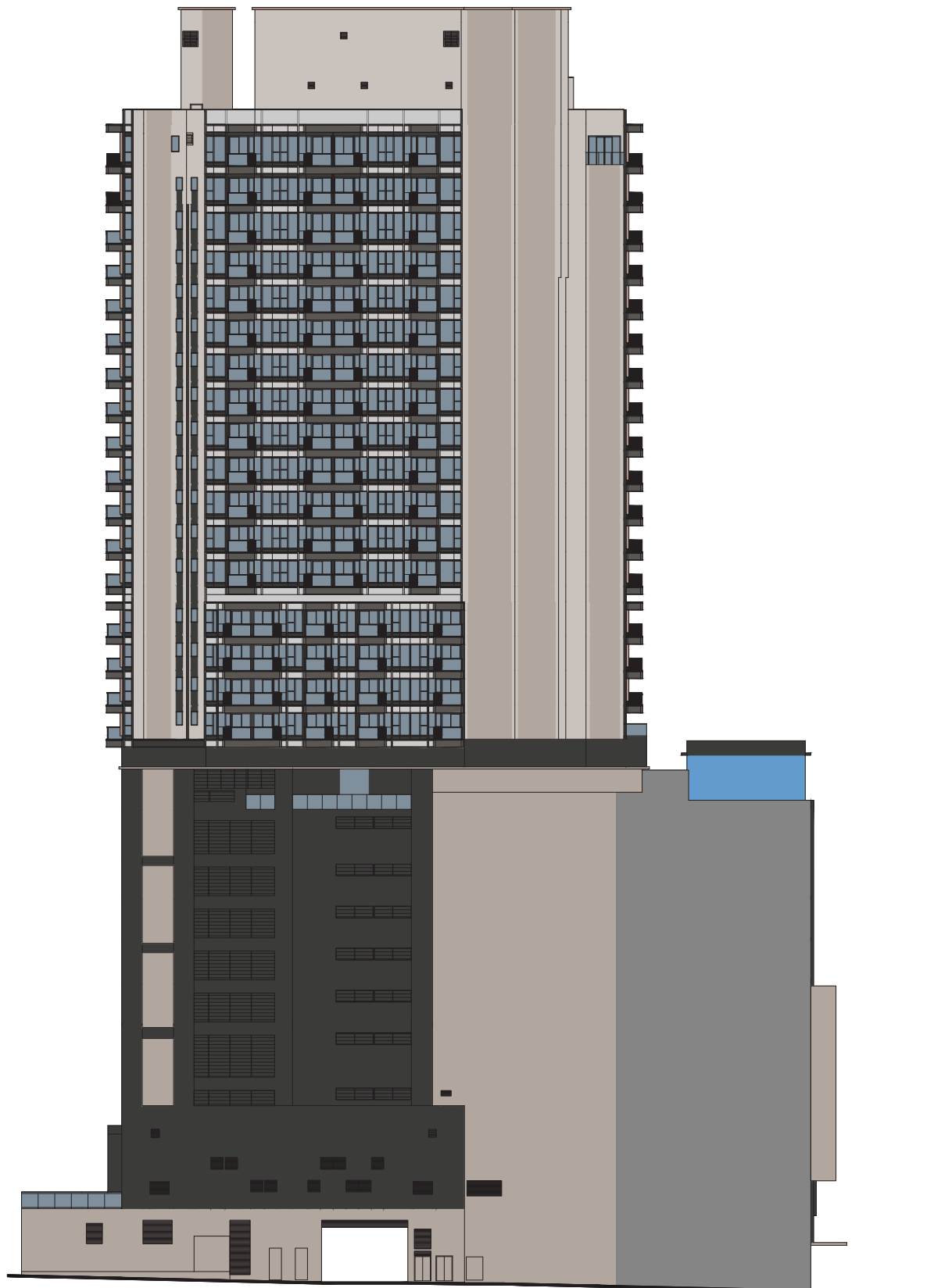
ELEVATION 3 立面 3
