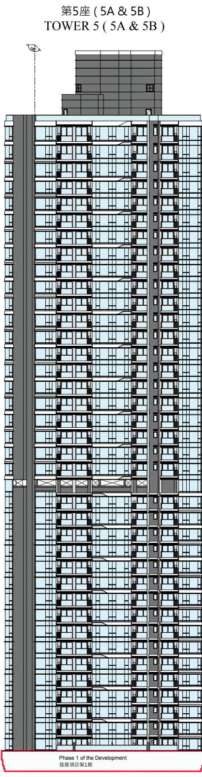
ELEVATION 2 立面圖 2
