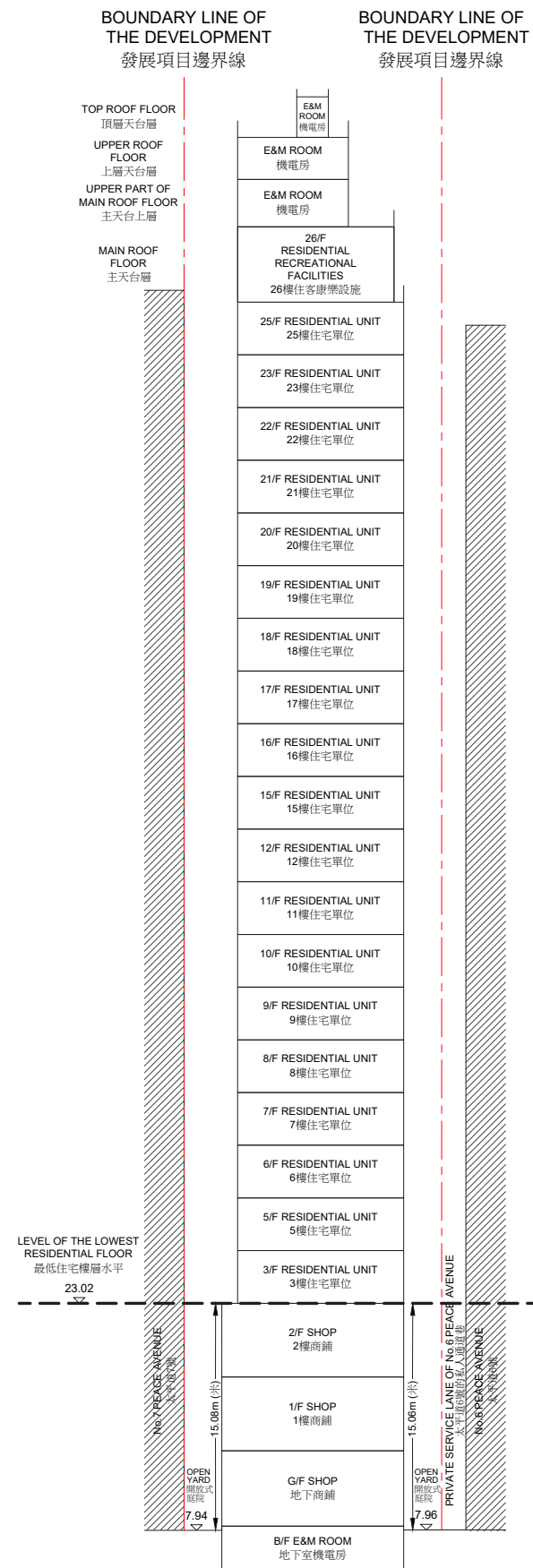
CROSS SECTION B-B 橫截面圖 B-B
