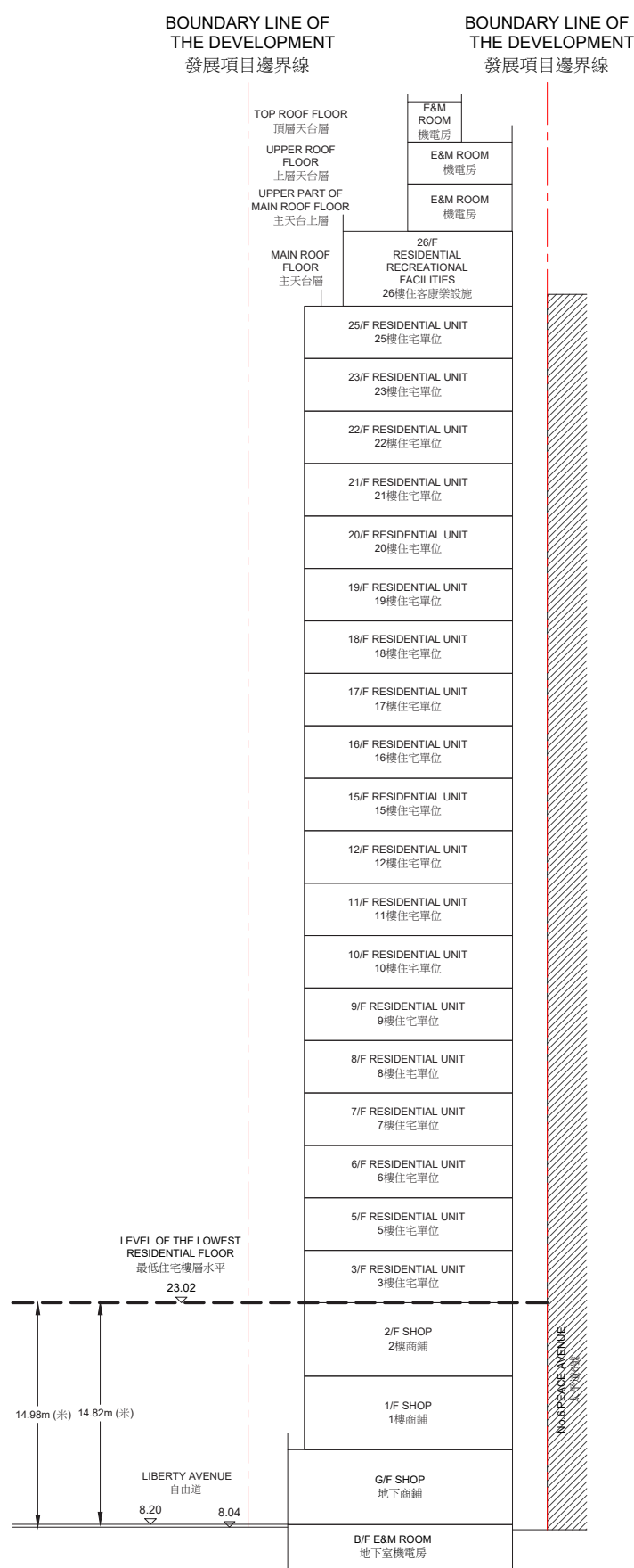
CROSS SECTION A-A 橫截面圖 A-A
