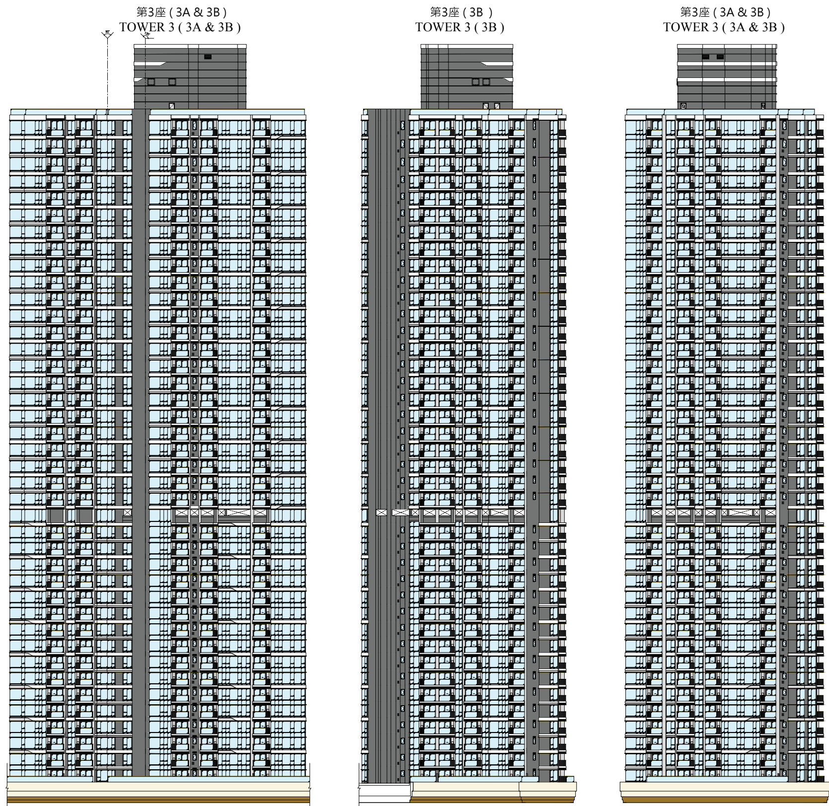
ELEVATION 1
