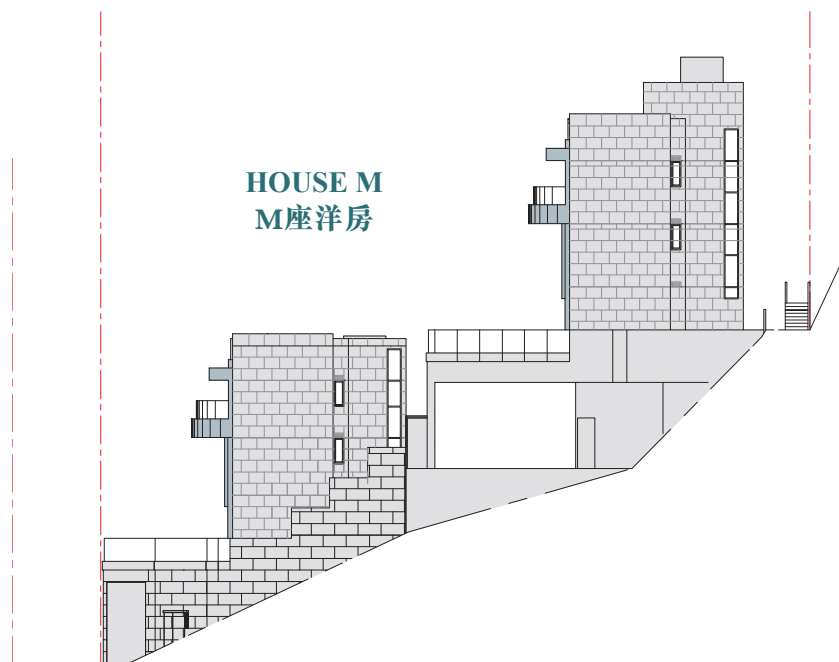
Elevation 4 立面圖 4
