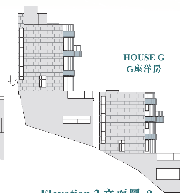
Elevation 2 立面圖 2
