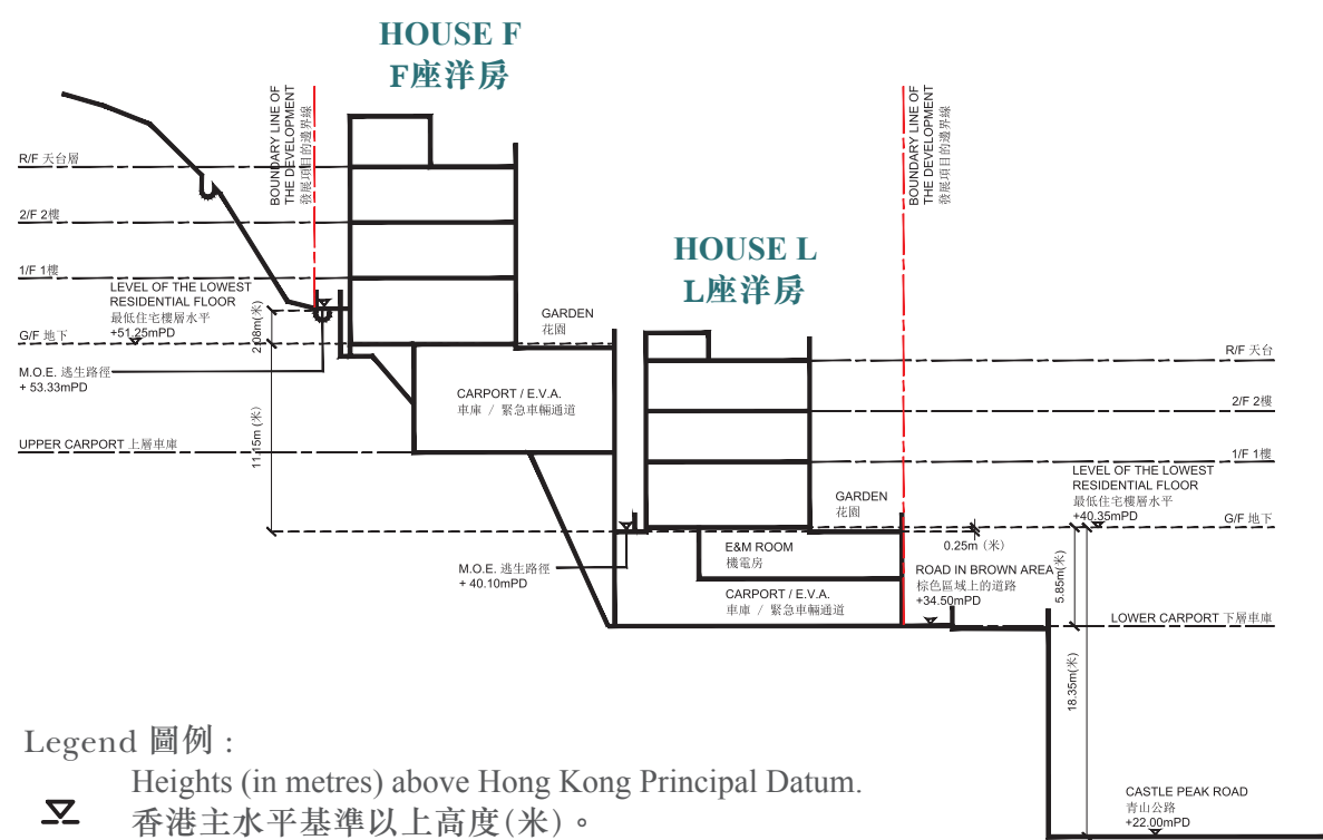
Cross - Section Plan H - H 橫截面圖 H-H HOUSE F F座洋房
