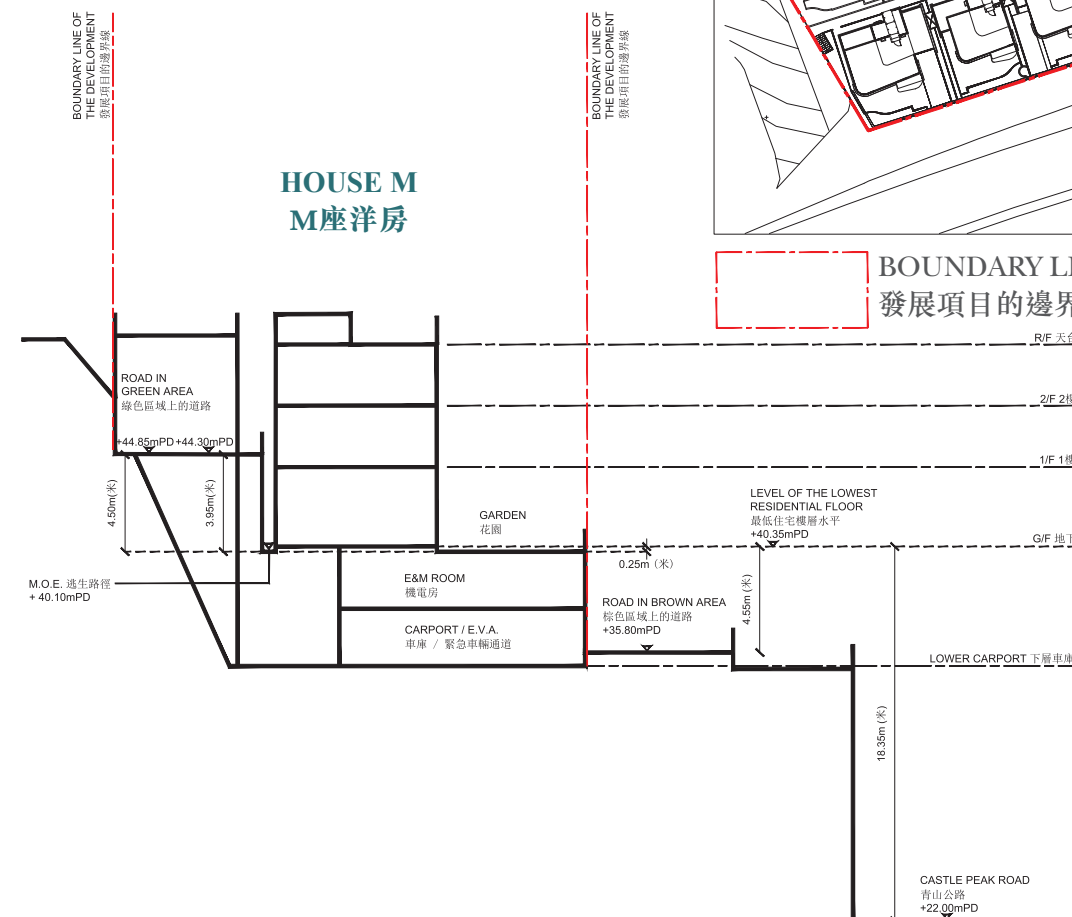
Cross - Section Plan I - I 橫截面圖 I-I
