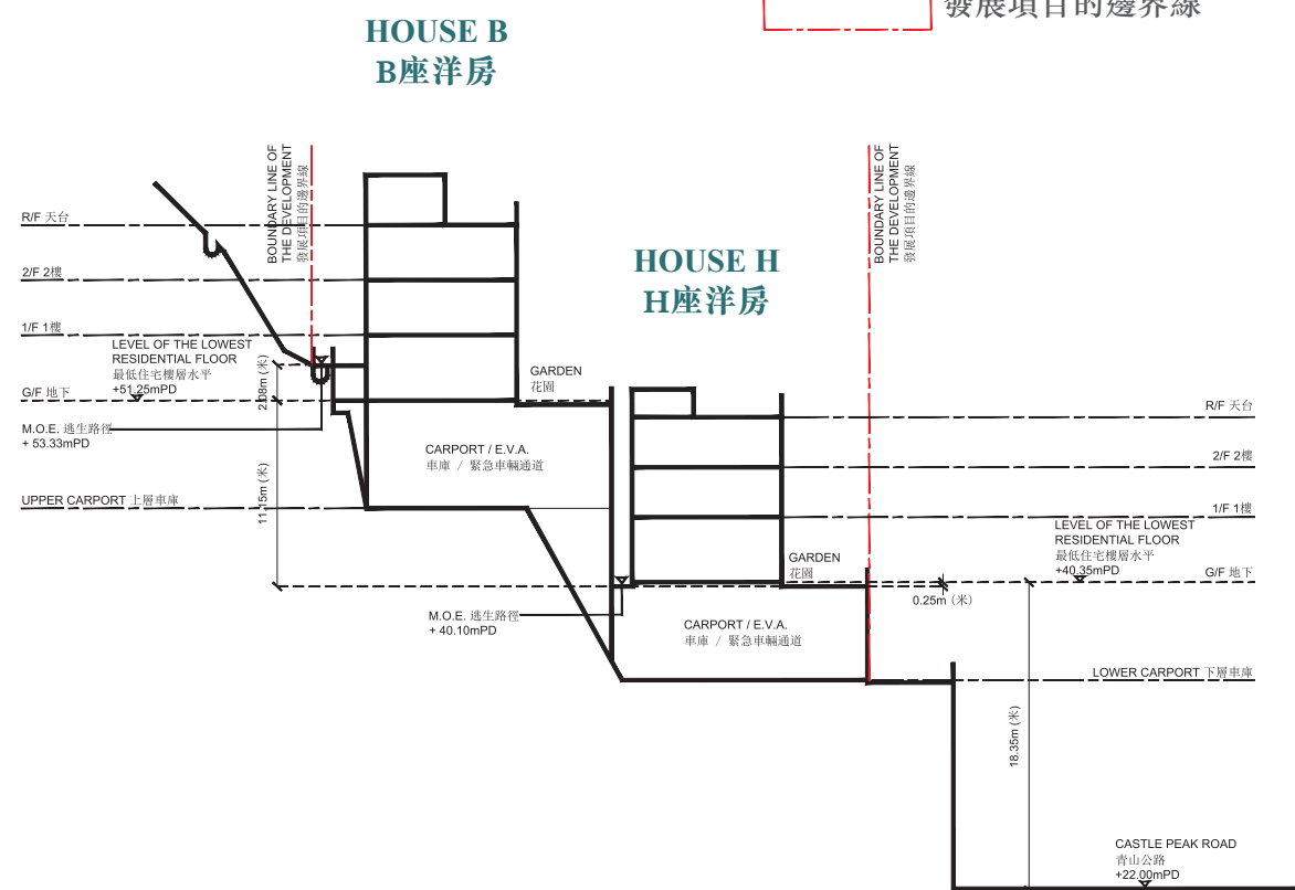
Cross - Section Plan D - D 橫截面圖 D-D
