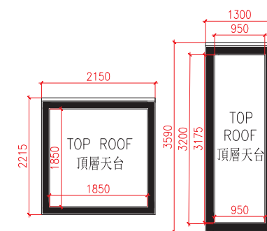
Top R/F For House I I座洋房頂層天台
