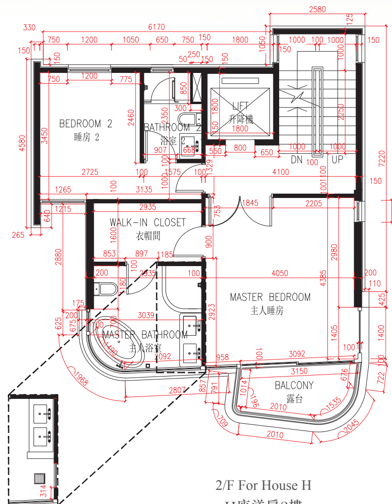
As-is Part Plan of 2/F 2樓現狀部分平面圖
