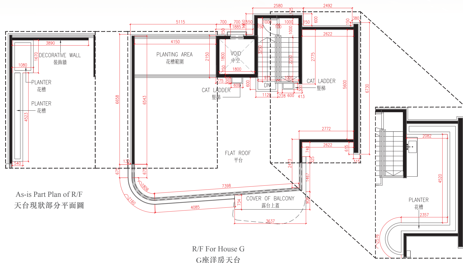
As-is Part Plan of R/F 天台現狀部分平面圖
