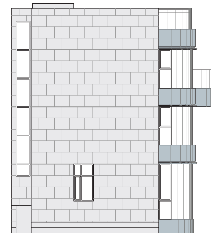
House G - ELEVATION 3 G座洋房 - 立面圖 3
