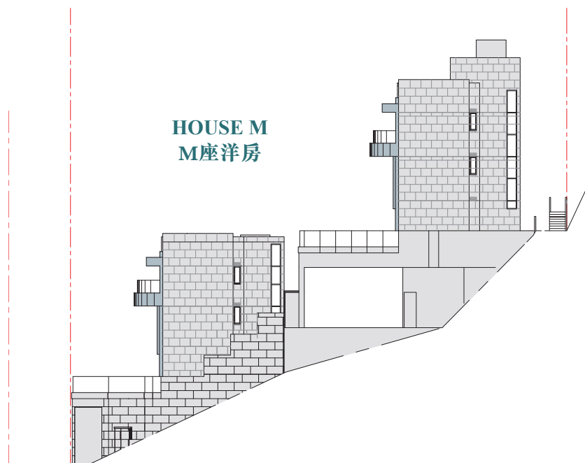
Elevation 4 立面圖 4
