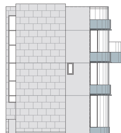
House L - ELEVATION 3 L座洋房 - 立面圖 3
