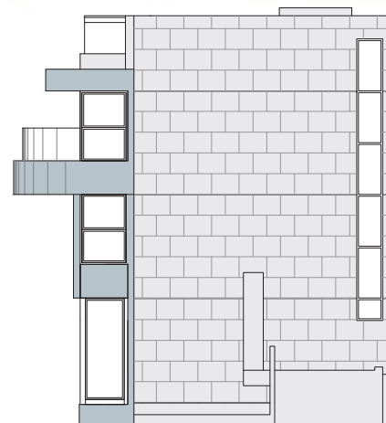
House I - ELEVATION 2 I座洋房 - 立面圖 2
