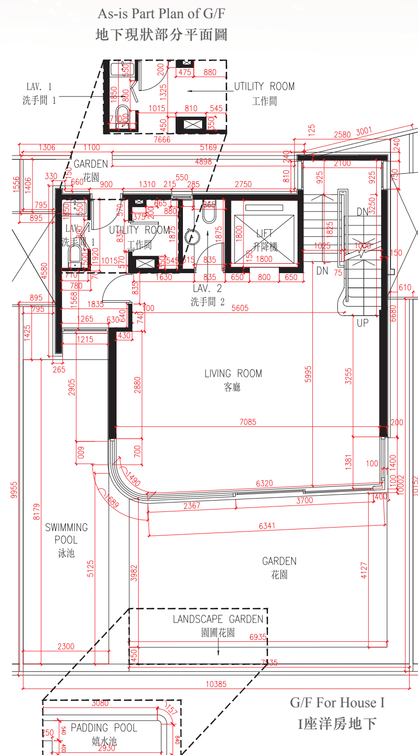
As-is Part Plan of G/F 地下現狀部分平面圖
