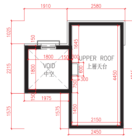
Upper R/F For House D D座洋房上層天台
