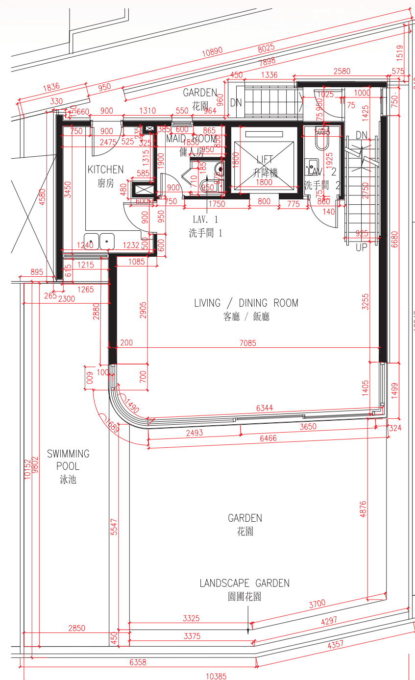
G/F For House J J座洋房地下
