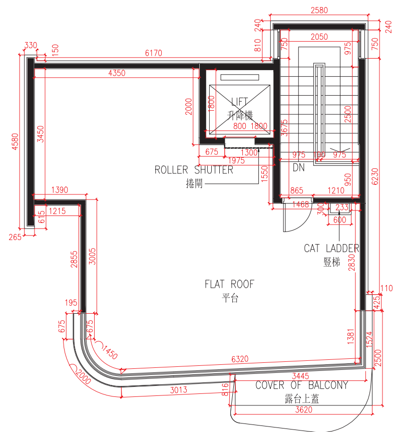
R/F For House B B座洋房天台
