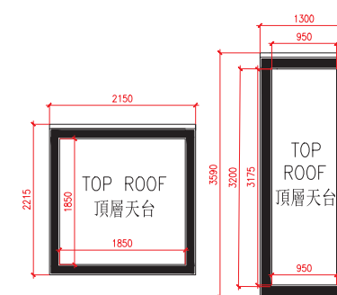
Top R/F For House K K座洋房頂層天台
