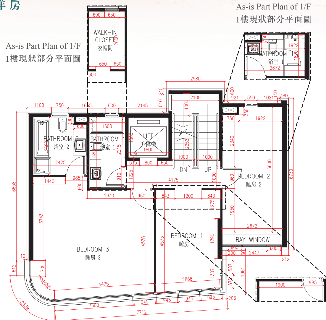
As-is Part Plan of 1/F 1樓現狀部分平面圖
