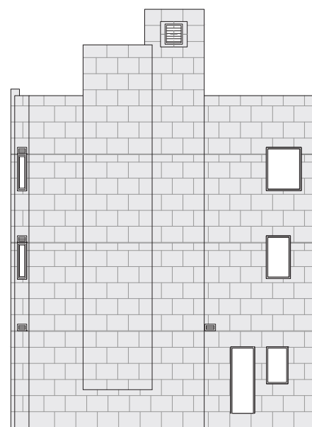
House F - ELEVATION 1 F座洋房 - 立面圖 1
