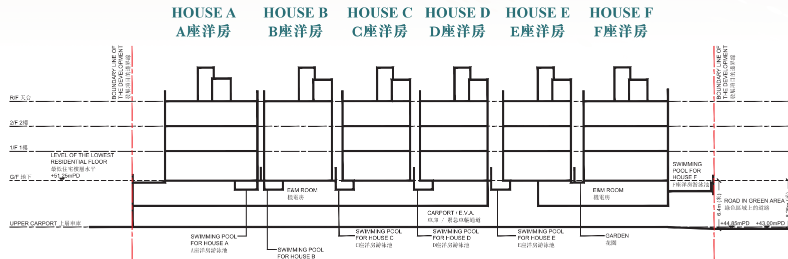
Cross - Section Plan A - A 橫截面圖 A-A
