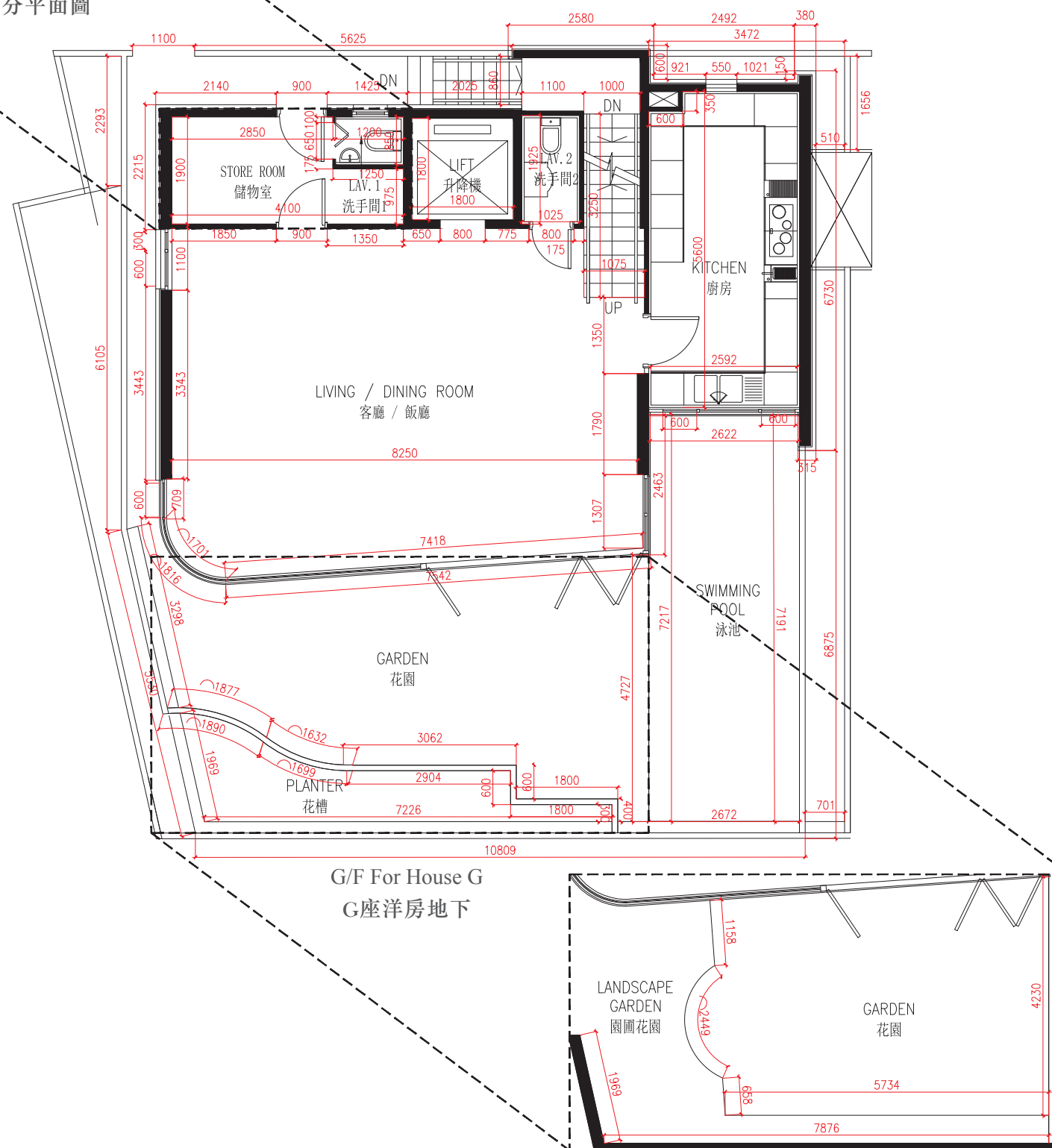
As-is Part Plan of G/F 地下現狀部分平面圖
