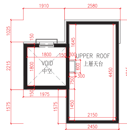
Upper R/F For House B B座洋房上層天台
