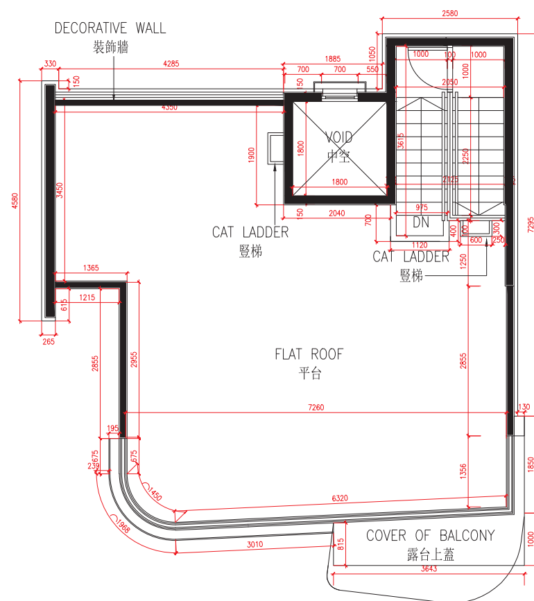
R/F For House K K座洋房天台
