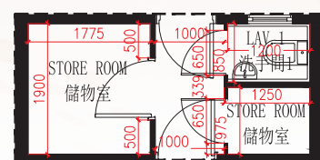
As-is Part Plan of G/F 地下現狀部分平面圖
