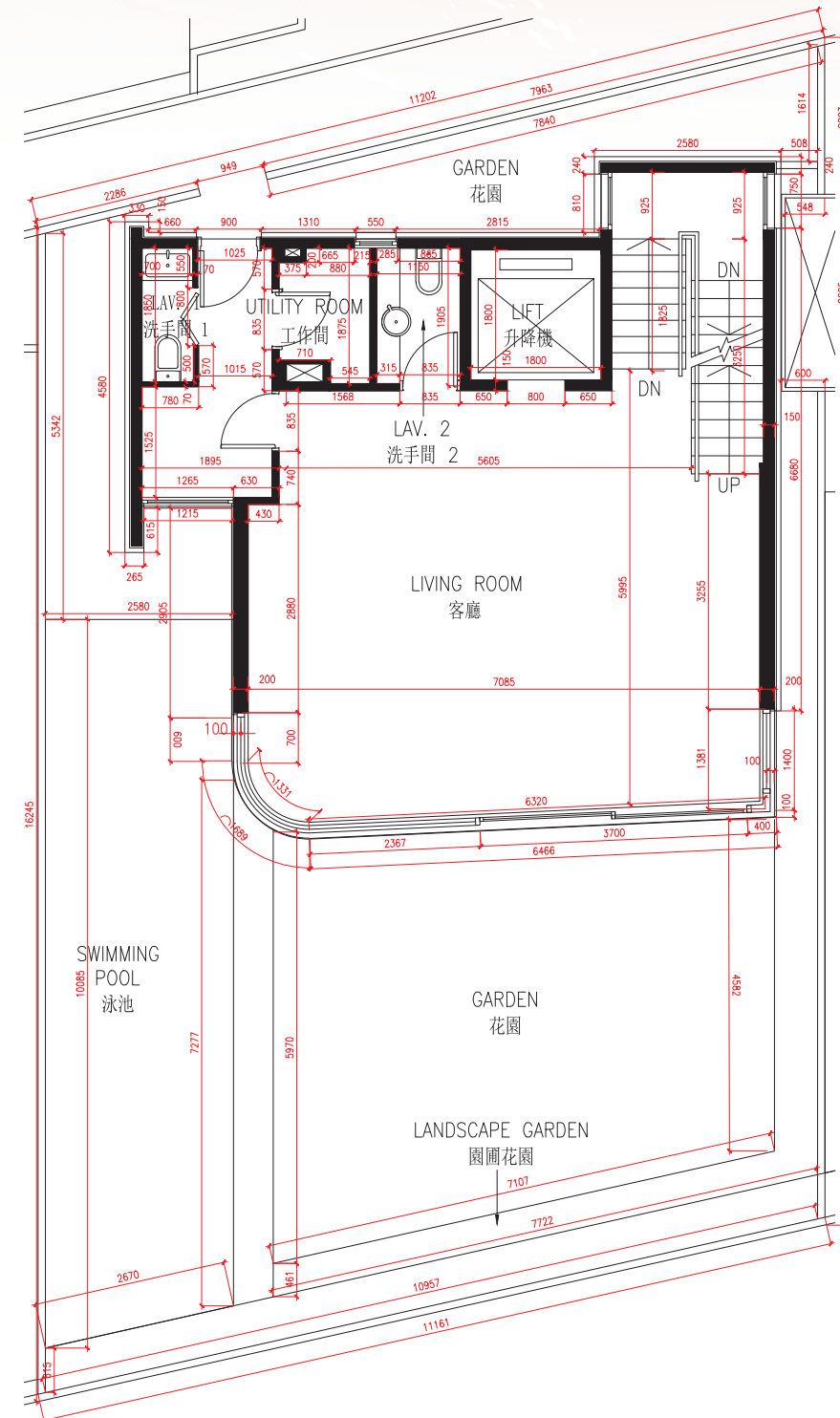
G/F For House K K座洋房地下
