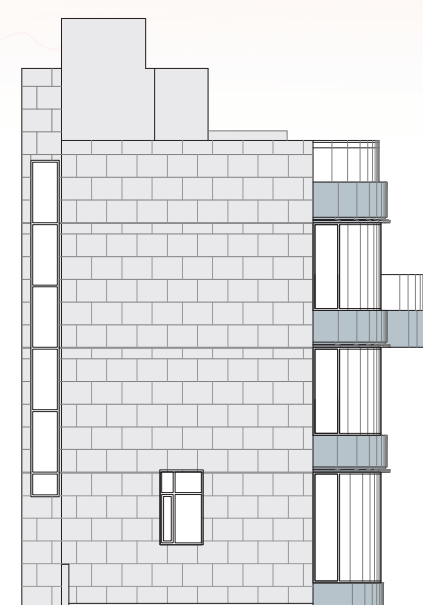
House A - ELEVATION 3 A座洋房 - 立面圖 3
