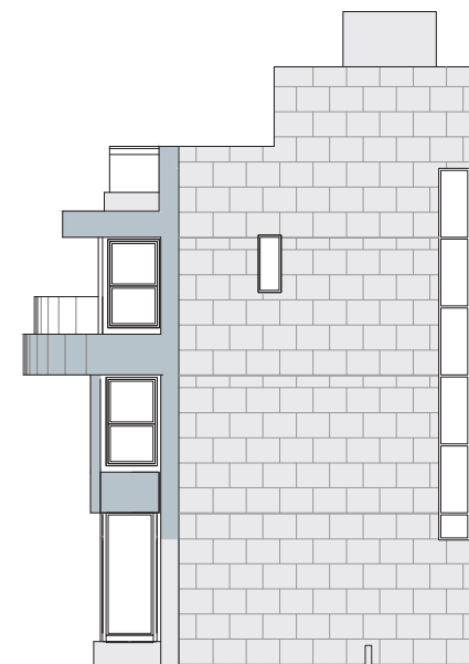
House D - ELEVATION 2 D座洋房 - 立面圖 2
