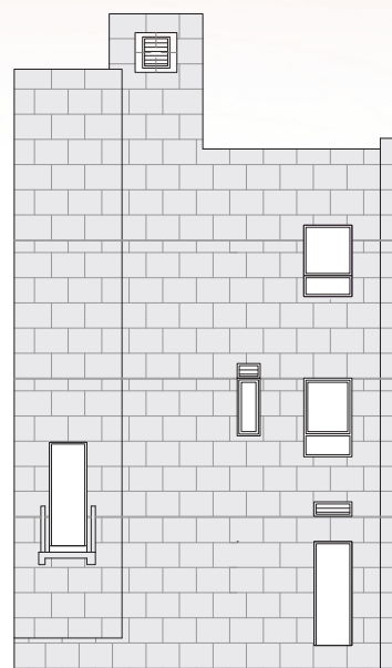
House E - ELEVATION 1 E座洋房 - 立面圖 1
