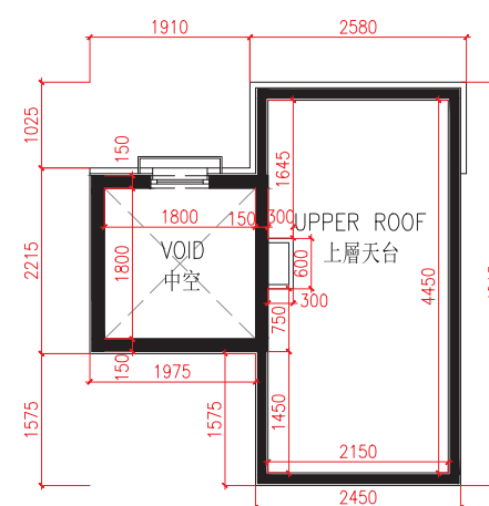
Upper R/F For House E E座洋房上層天台
