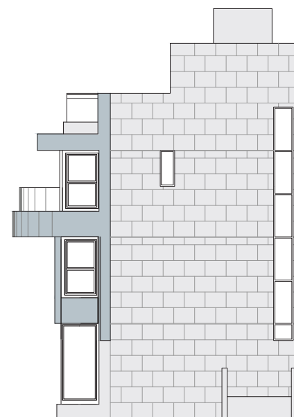
House B - ELEVATION 2 B座洋房 - 立面圖 2
