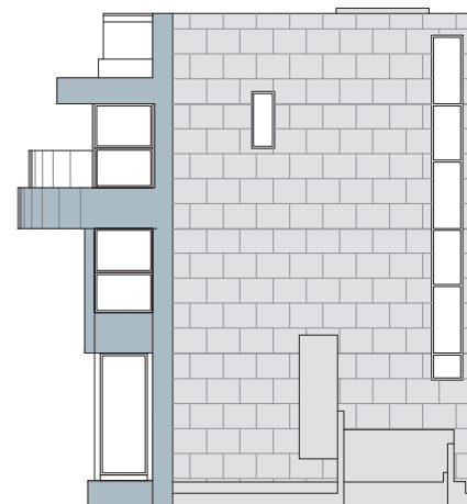
House K - ELEVATION 2 K座洋房 - 立面圖 2
