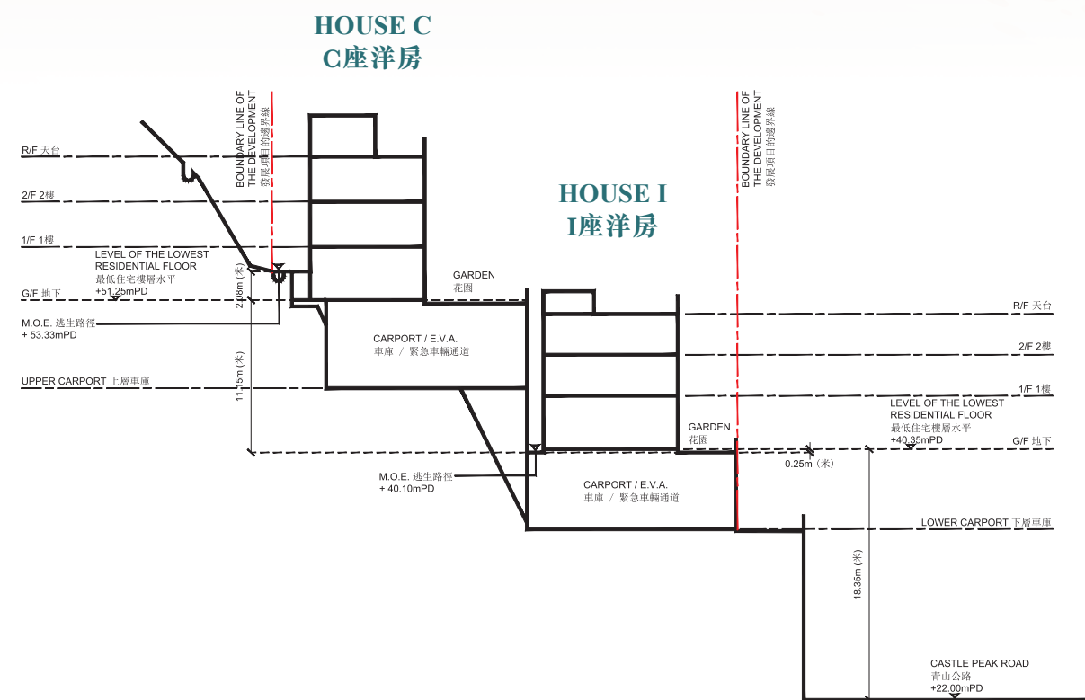
Cross - Section Plan E - E 橫截面圖 E-E
