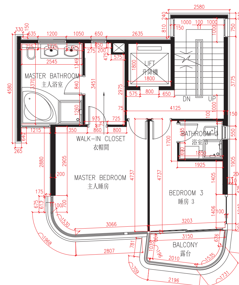
2/F For House J J座洋房2樓
