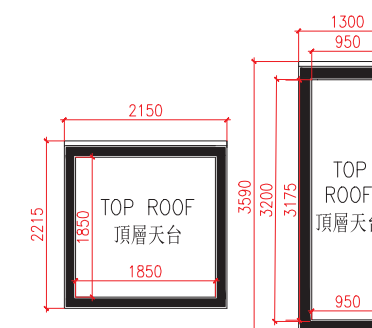
Top R/F For House M M座洋房頂層天台
