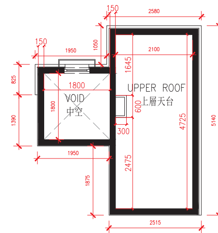
Upper R/F For House F F座洋房上層天台
