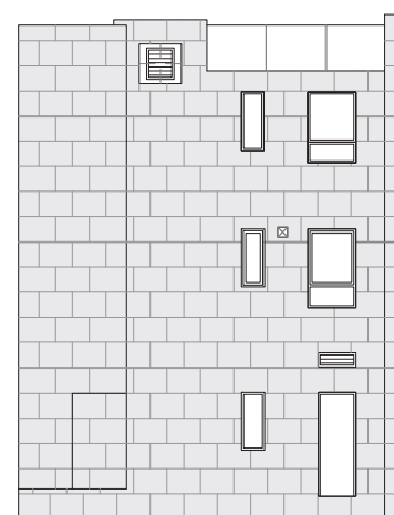
House J - ELEVATION 1 J座洋房 - 立面圖 1
