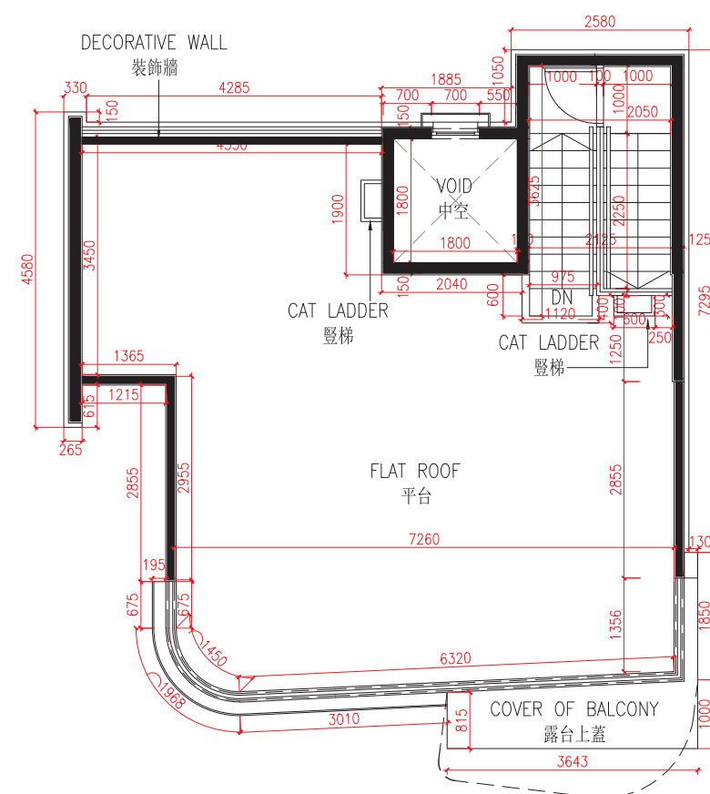
R/F For House J J座洋房天台
