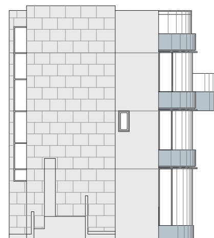
House H - ELEVATION 3 H座洋房 - 立面圖 3
