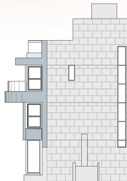
House E - ELEVATION 2 E座洋房 - 立面圖 2
