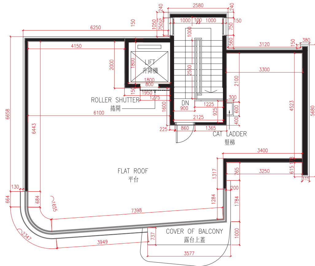
R/F For House A A座洋房天台
