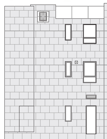
House I - ELEVATION 1 I座洋房 - 立面圖 1
