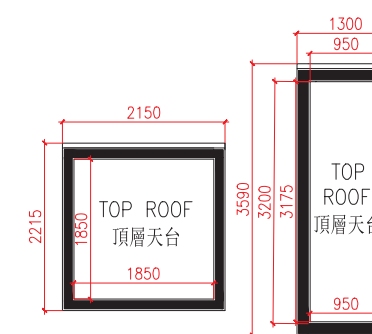
Top R/F For House I I座洋房頂層天台
