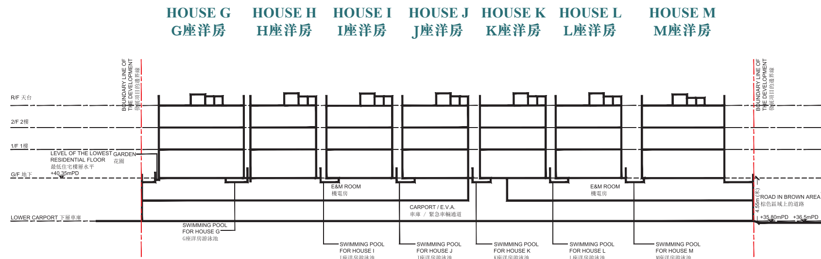
Cross - Section Plan B - B 橫截面圖 B-B
