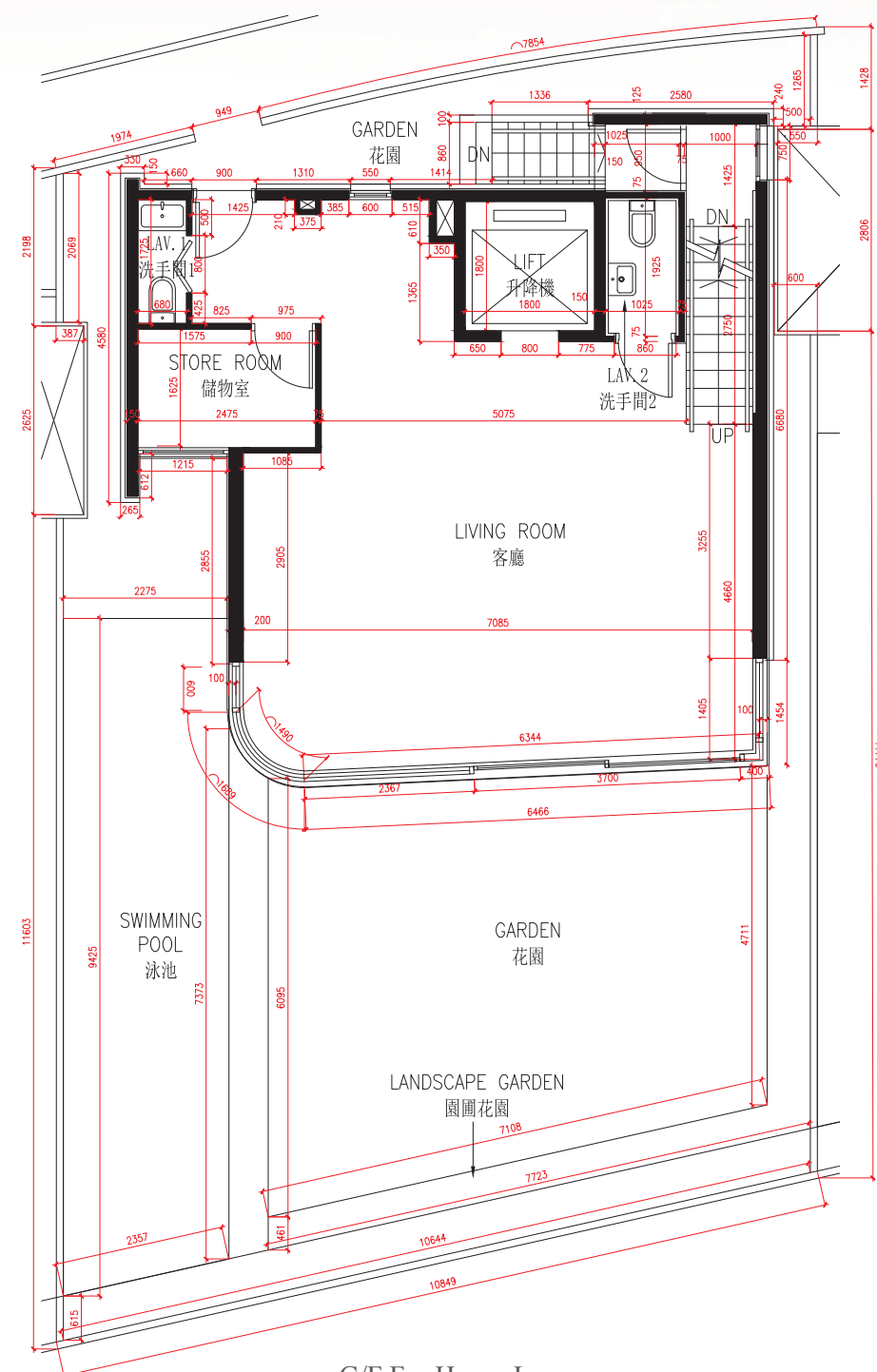
G/F For House L L座洋房地下
