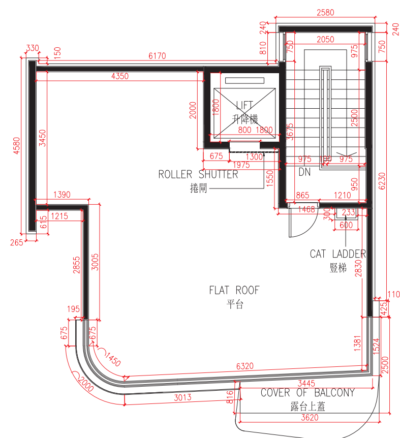
R/F For House C C座洋房天台
