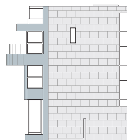
House H - ELEVATION 2 H座洋房 - 立面圖 2
