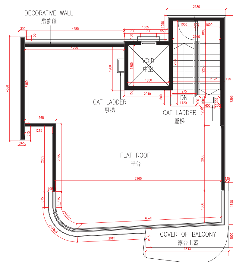
R/F For House L L座洋房天台
