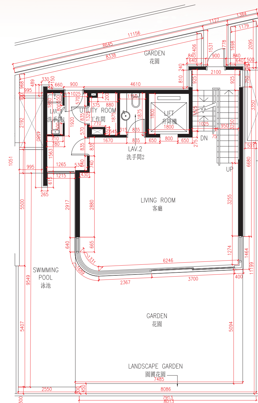
G/F For House B B座洋房地下
