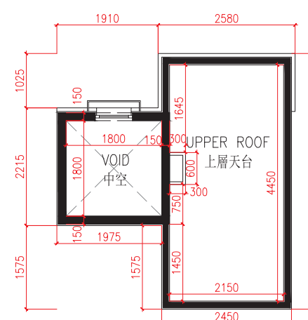
Upper R/F For House C C座洋房上層天台
