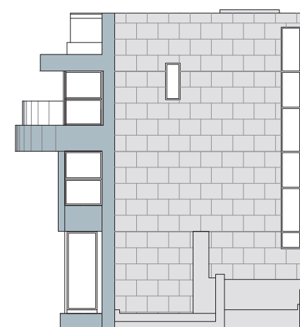
House L - ELEVATION 2 L座洋房 - 立面圖 2
