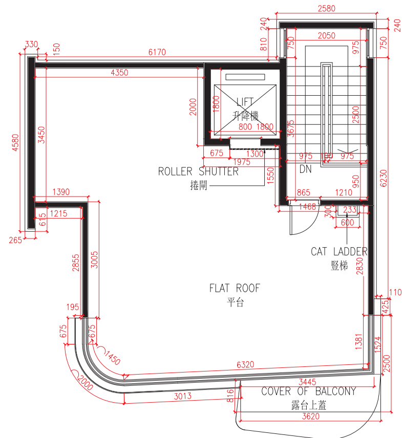
R/F For House D D座洋房天台
