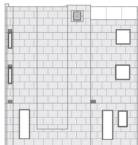
House M - ELEVATION 1 M座洋房 - 立面圖 1
