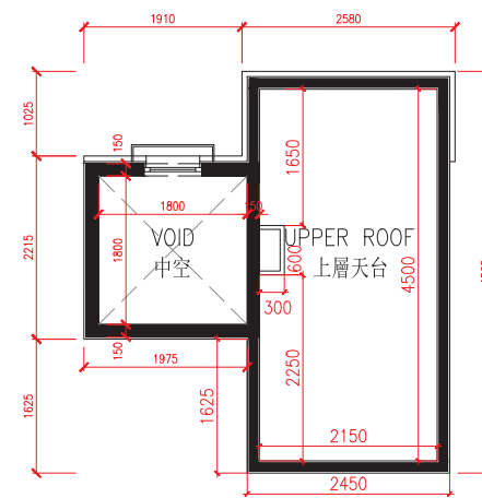
Upper R/F For House A A座洋房上層天台
