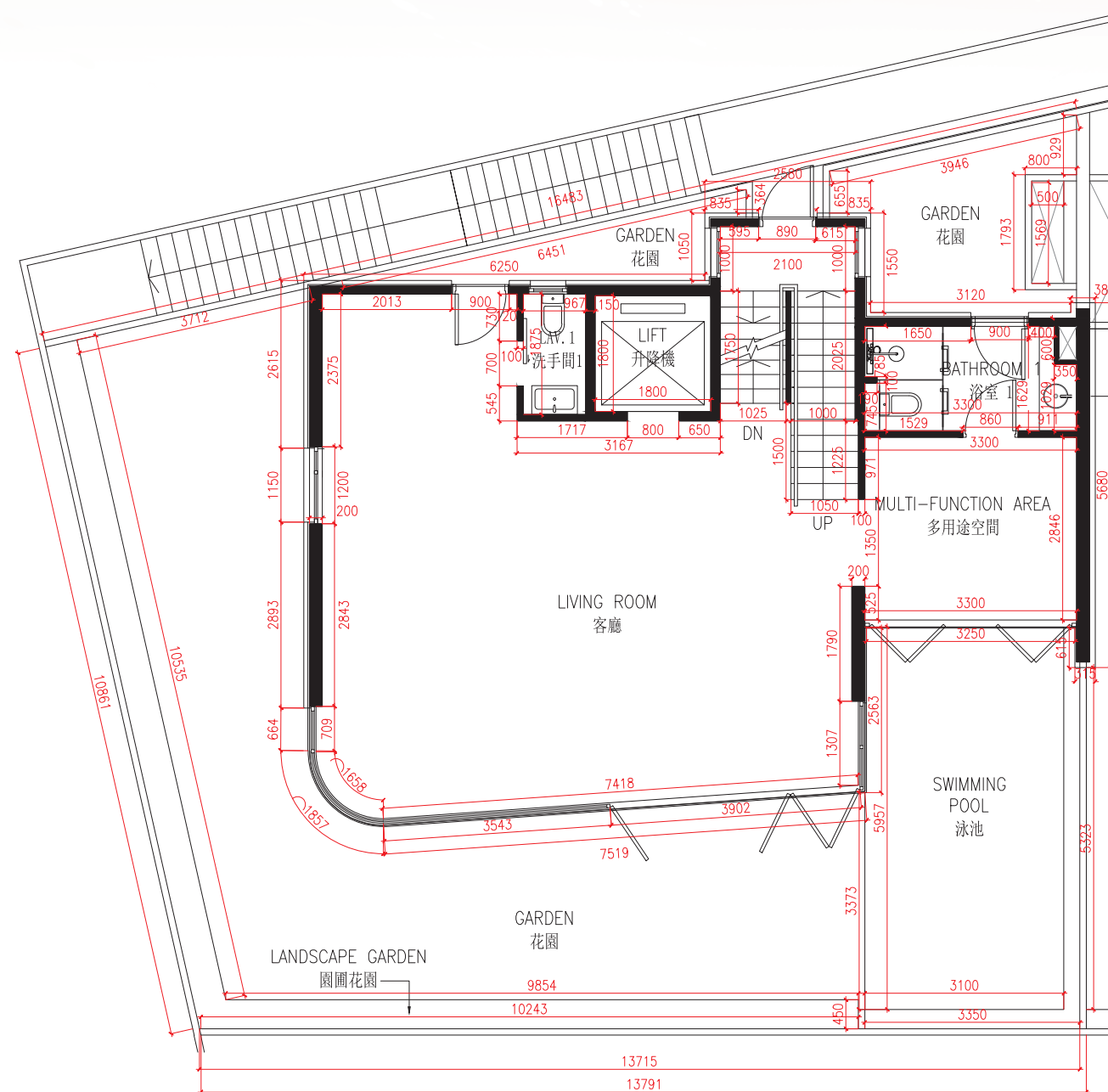
G/F For House A A座洋房地下
