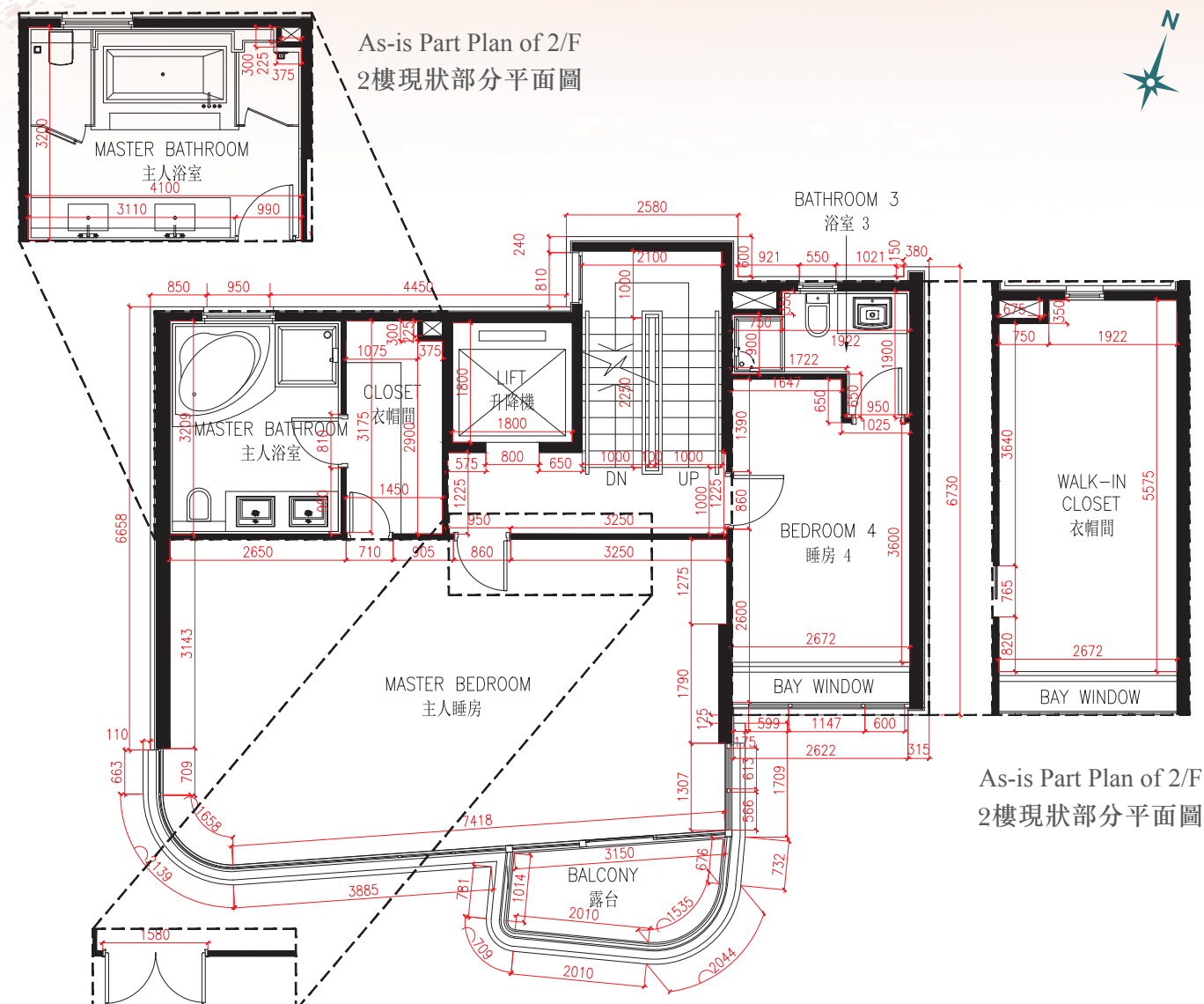
As-is Part Plan of 2/F 2樓現狀部分平面圖
