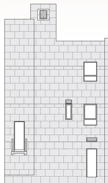
House C - ELEVATION 1 C座洋房 - 立面圖 1
