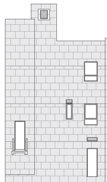
House B - ELEVATION 1 B座洋房 - 立面圖 1
