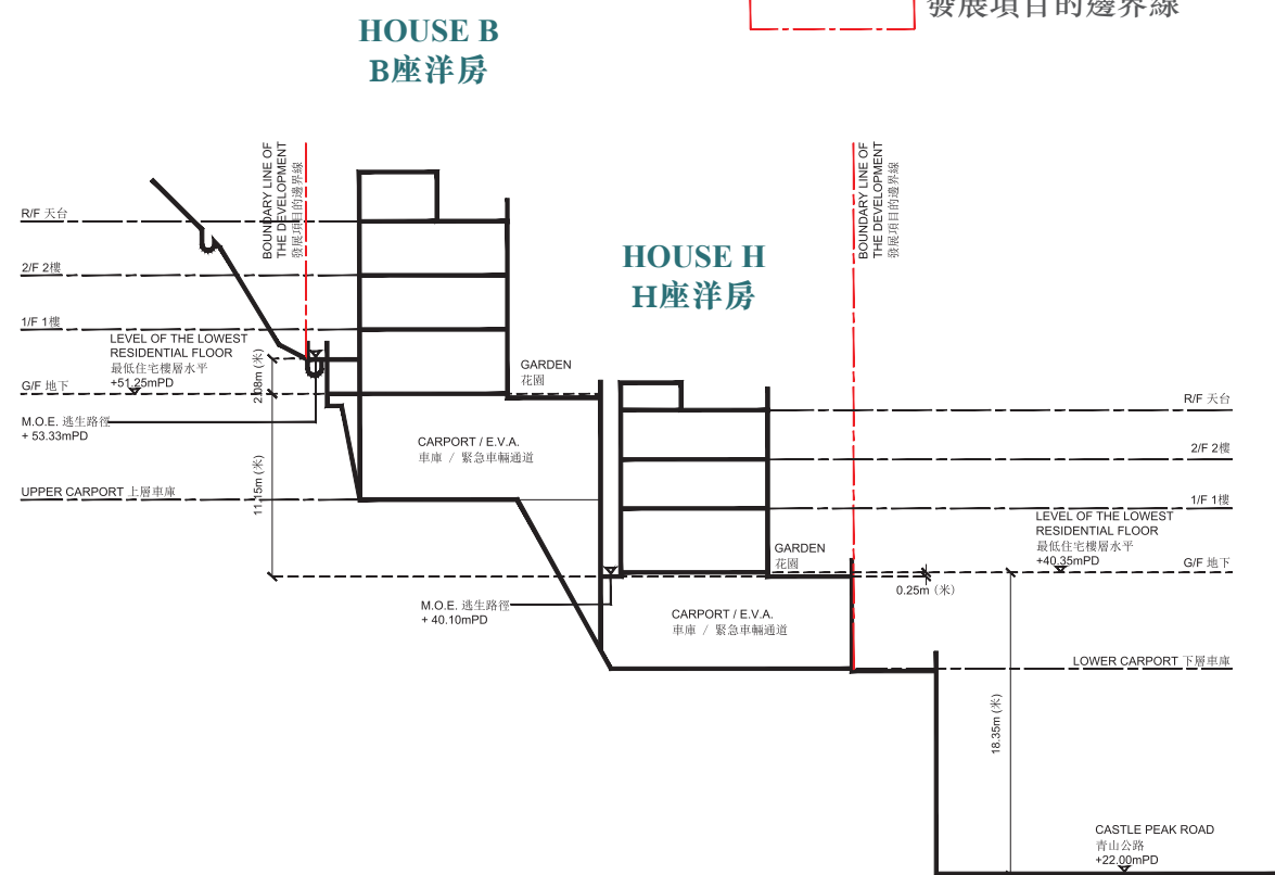
Cross - Section Plan D - D 橫截面圖 D-D
