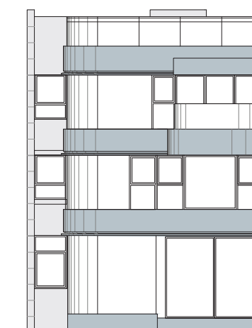
House L - ELEVATION 4 L座洋房 - 立面圖 4
