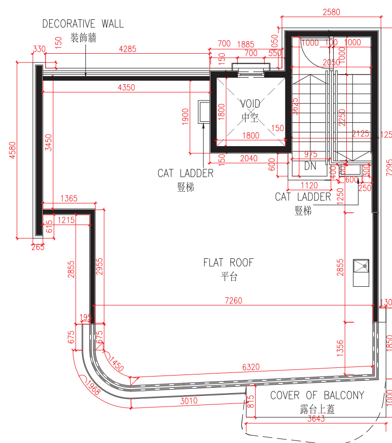
R/F For House I I座洋房天台
