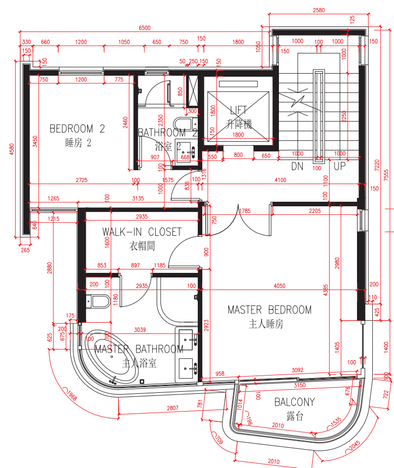
2/F For House L L座洋房2樓
