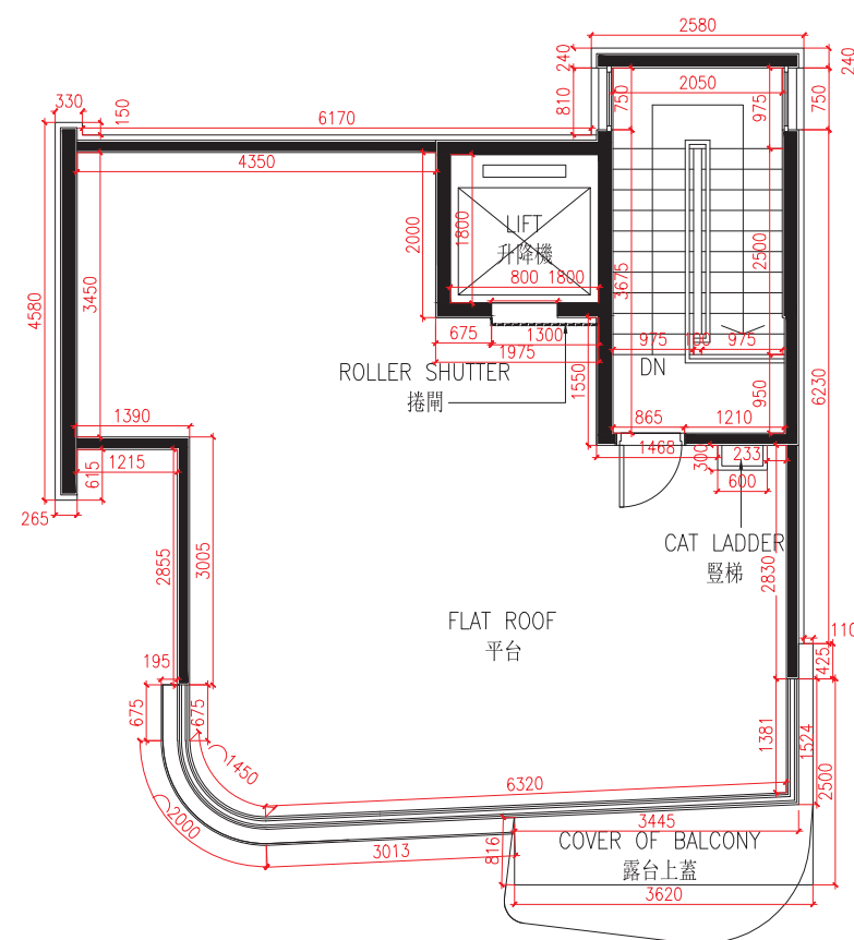
R/F For House E E座洋房天台
