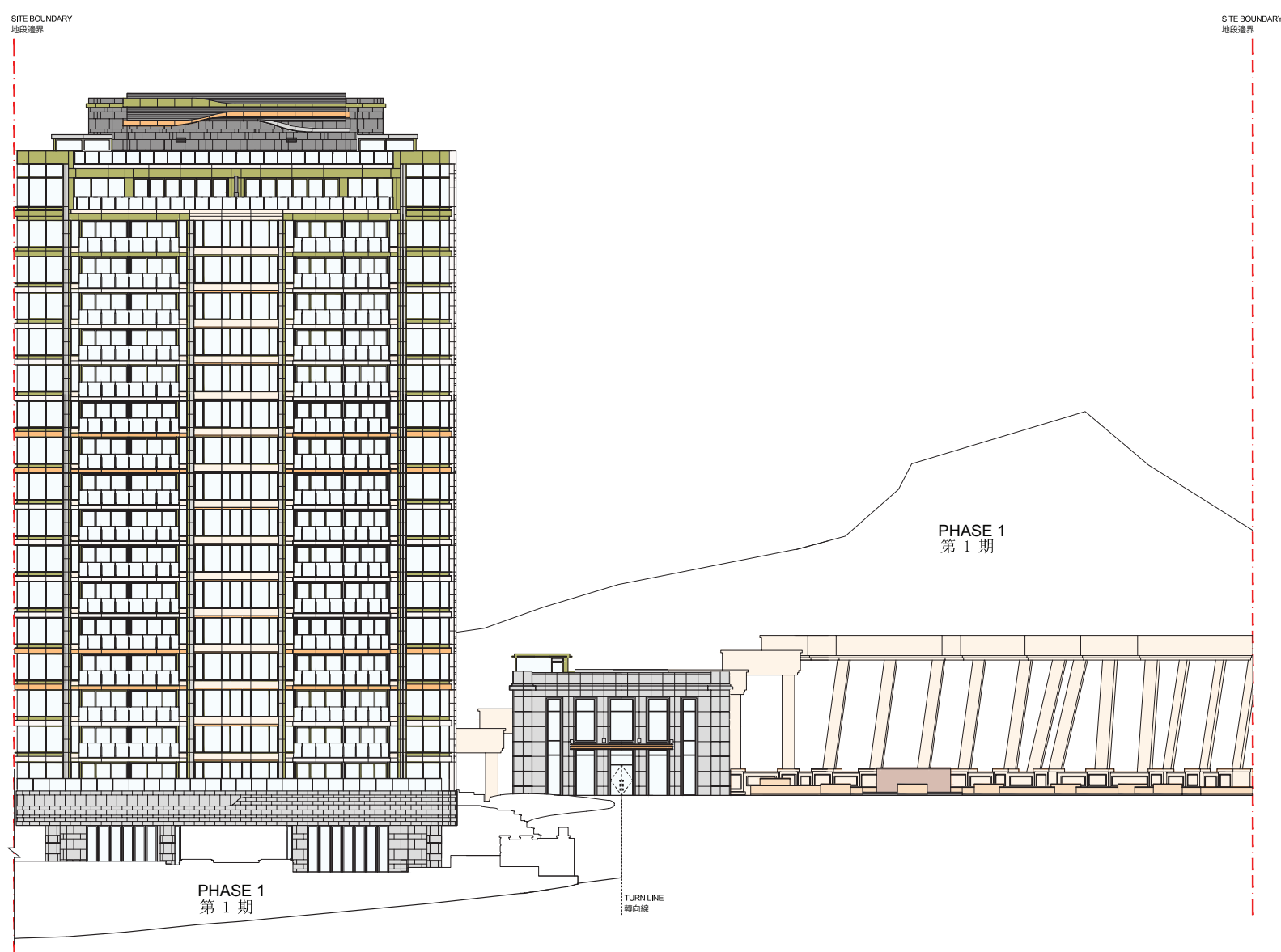
立面圖1 Elevation 1
