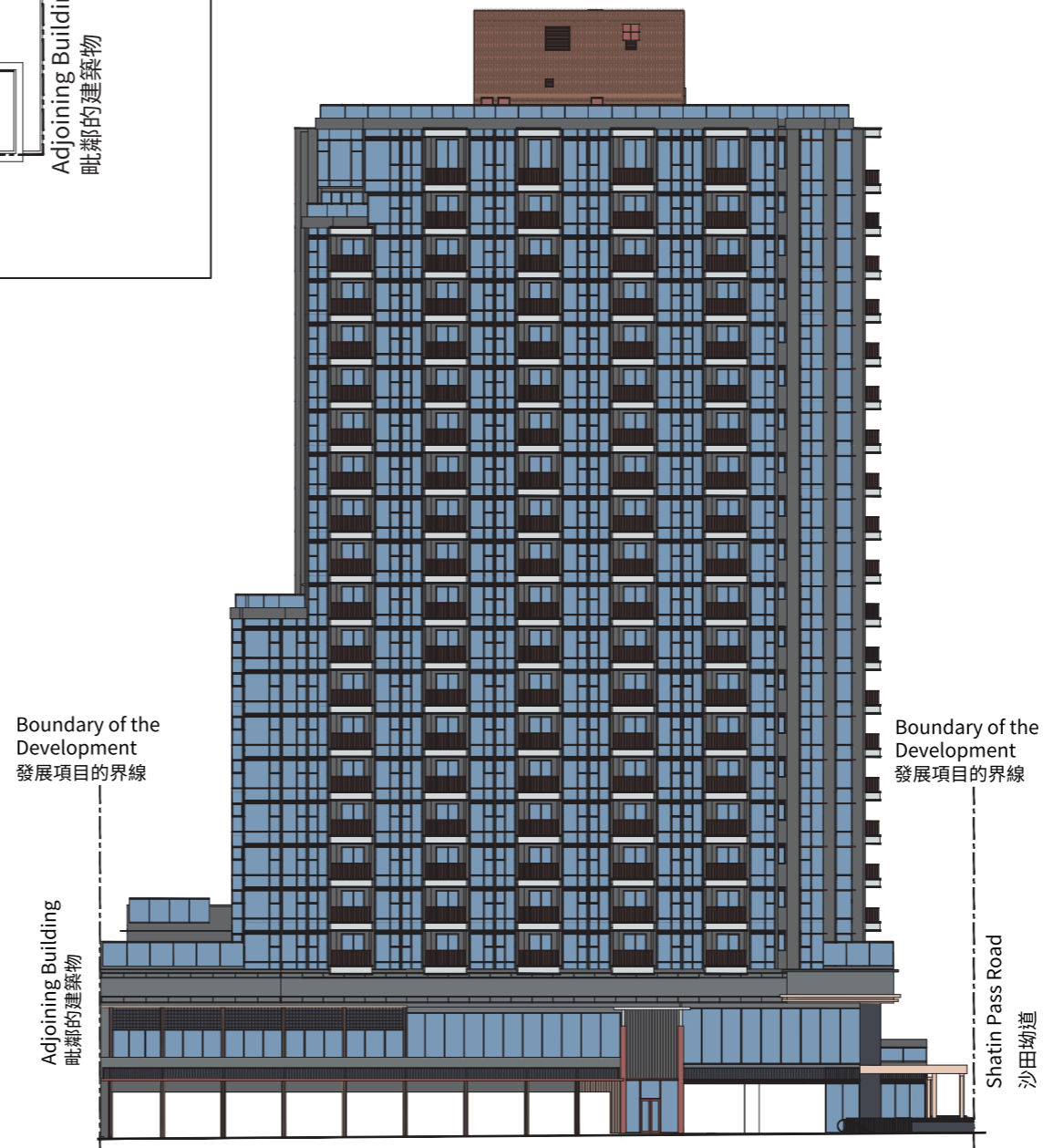
Elevation A A 立面圖
