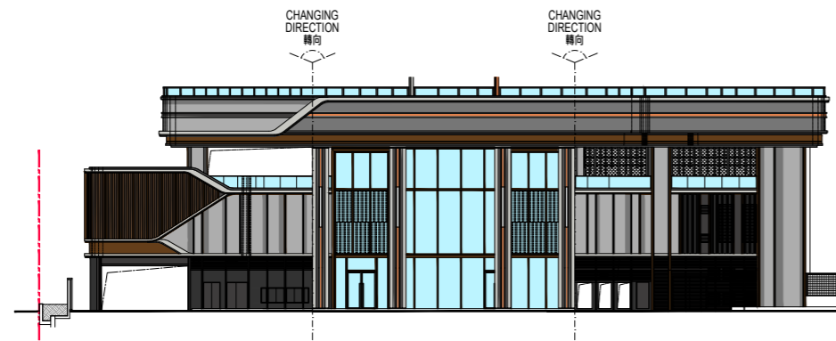
ELEVATION E 立面圖 E
