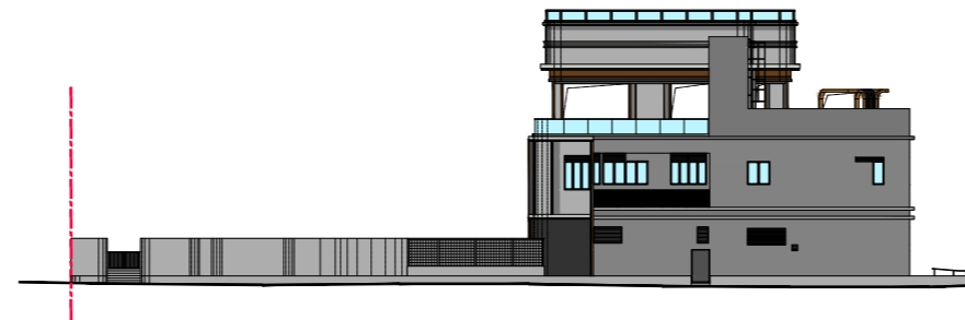
ELEVATION G 立面圖 G
