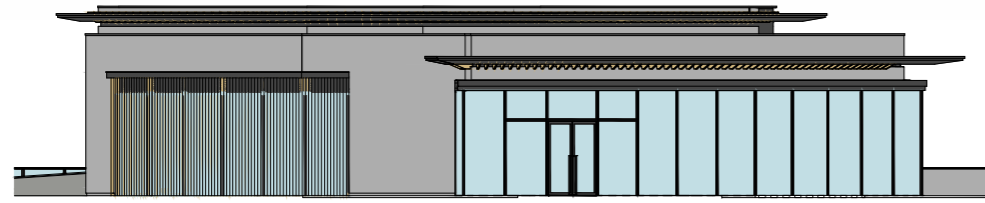
ELEVATION PLAN 1 立面圖 1
