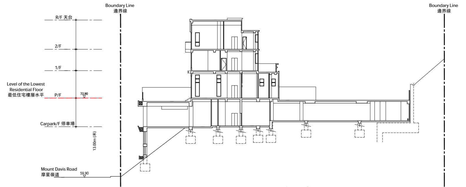
Cross-Section Plan of House D 洋房 D 截面圖
