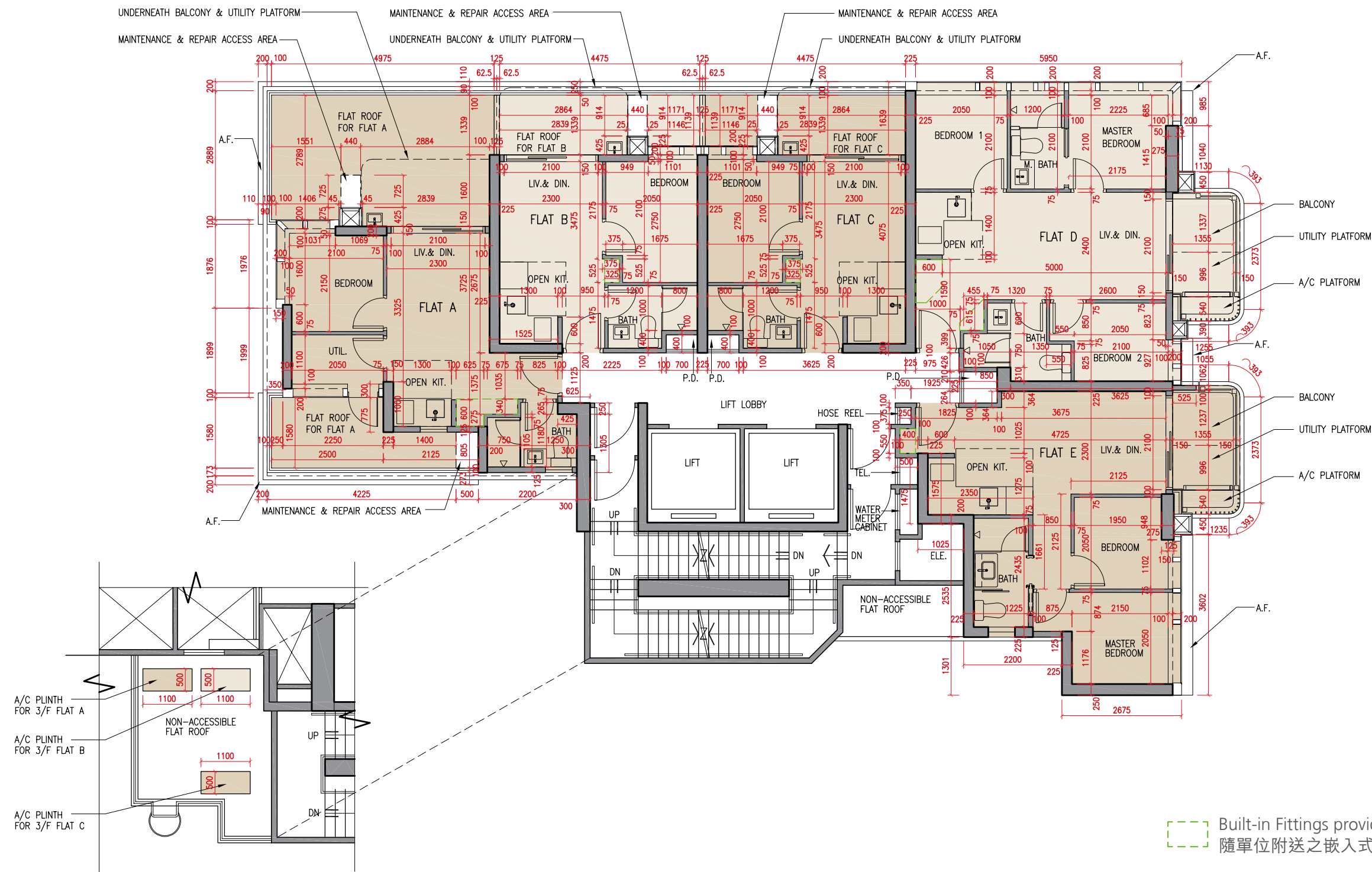
PART PLAN OF FLAT ROOF AT LEVEL 53.40 位於53.40水平的平台部分平面圖
