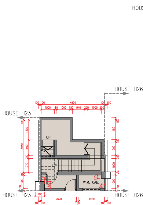
地庫平面圖 B/F Plan
