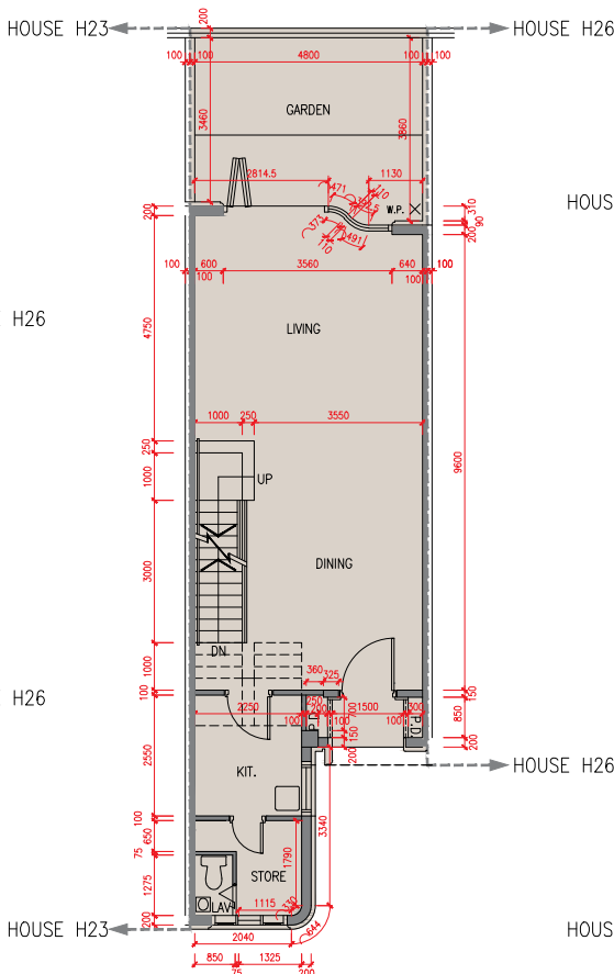
地下平面圖 G/F Plan
