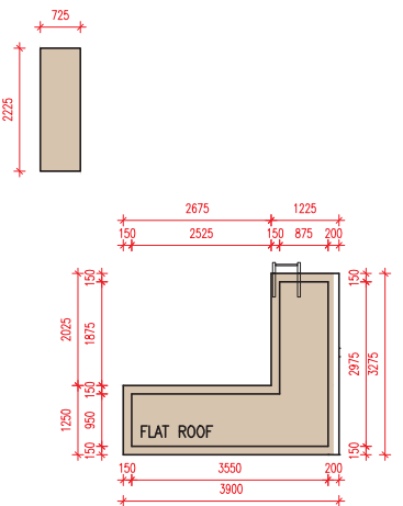
As-is Part Plan of ROOF/F (See Note E) 天台之部分現狀圖 (見備註戊)
