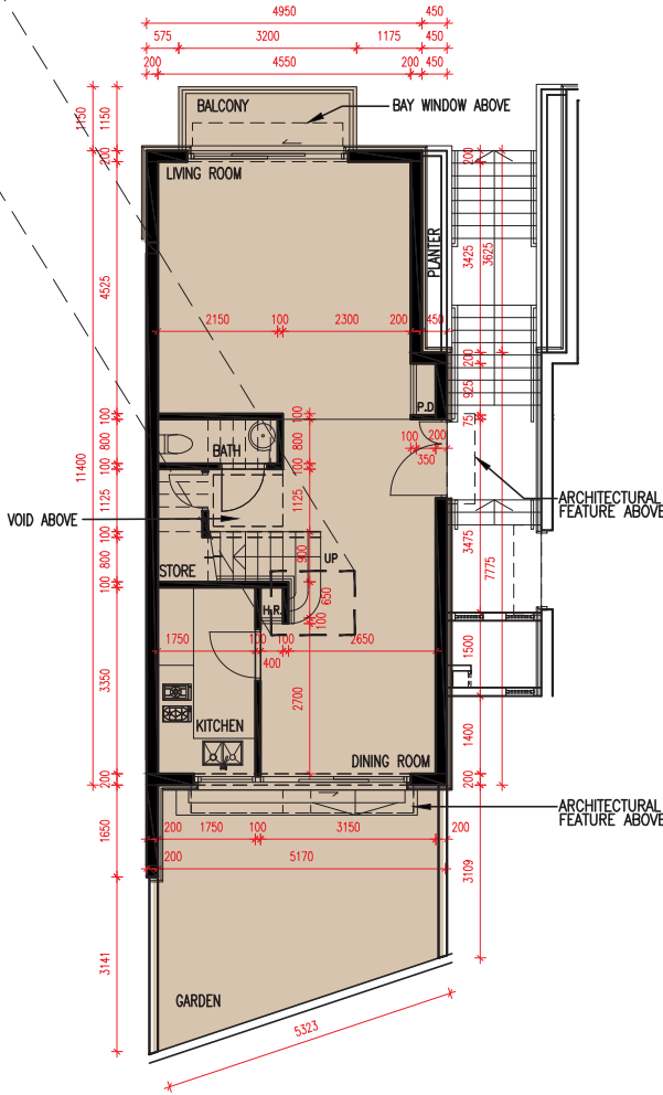
G/F PLAN 地面層平面圖
