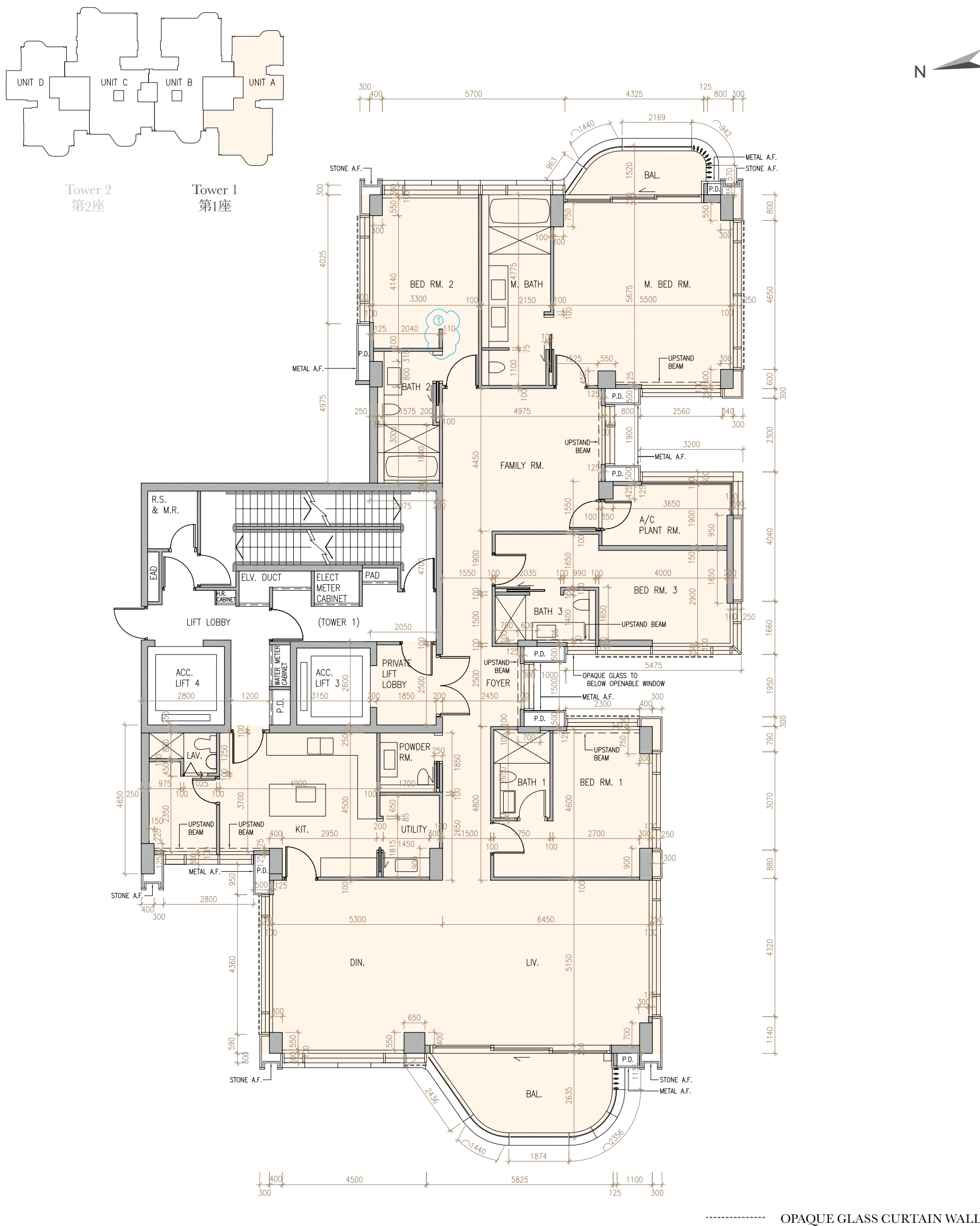
UNIT A 5/F - 12/F, 15/F AND 17/F FLOOR PLAN SHOWING LATEST LAYOUT A 單位 5樓 - 12樓、15樓及17樓現狀平面圖
