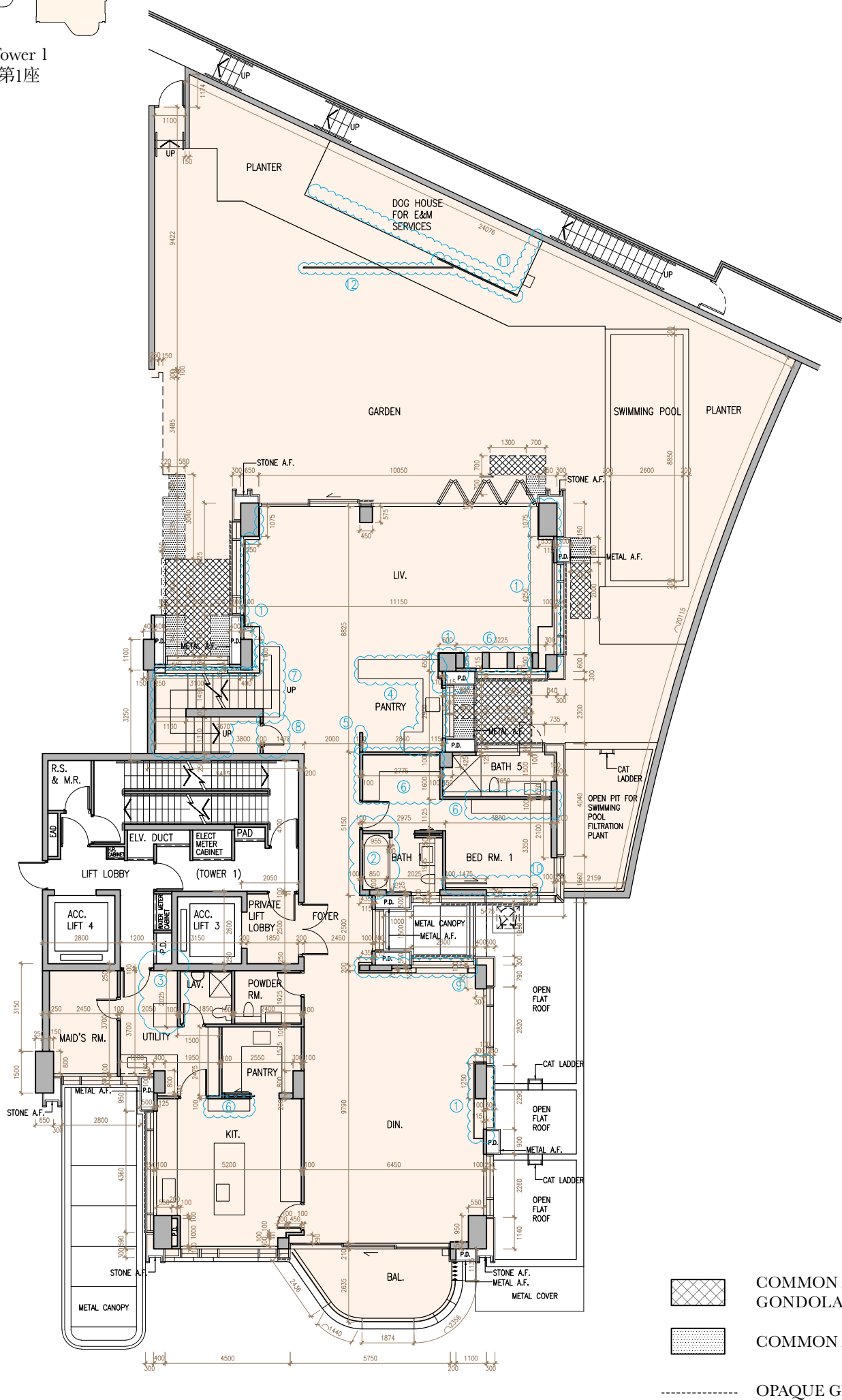
GARDEN UNIT A 1/F FLOOR PLAN SHOWING LATEST LAYOUT 花園單位 A 1樓現狀平面圖
