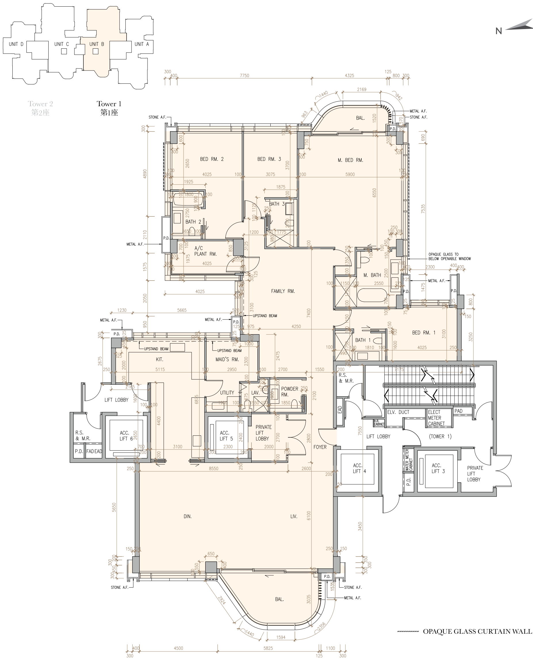
UNIT B 5/F - 12/F AND 16/F - 17/F FLOOR PLAN B 單位 5樓 - 12樓及16樓 - 17樓樓面平面圖
