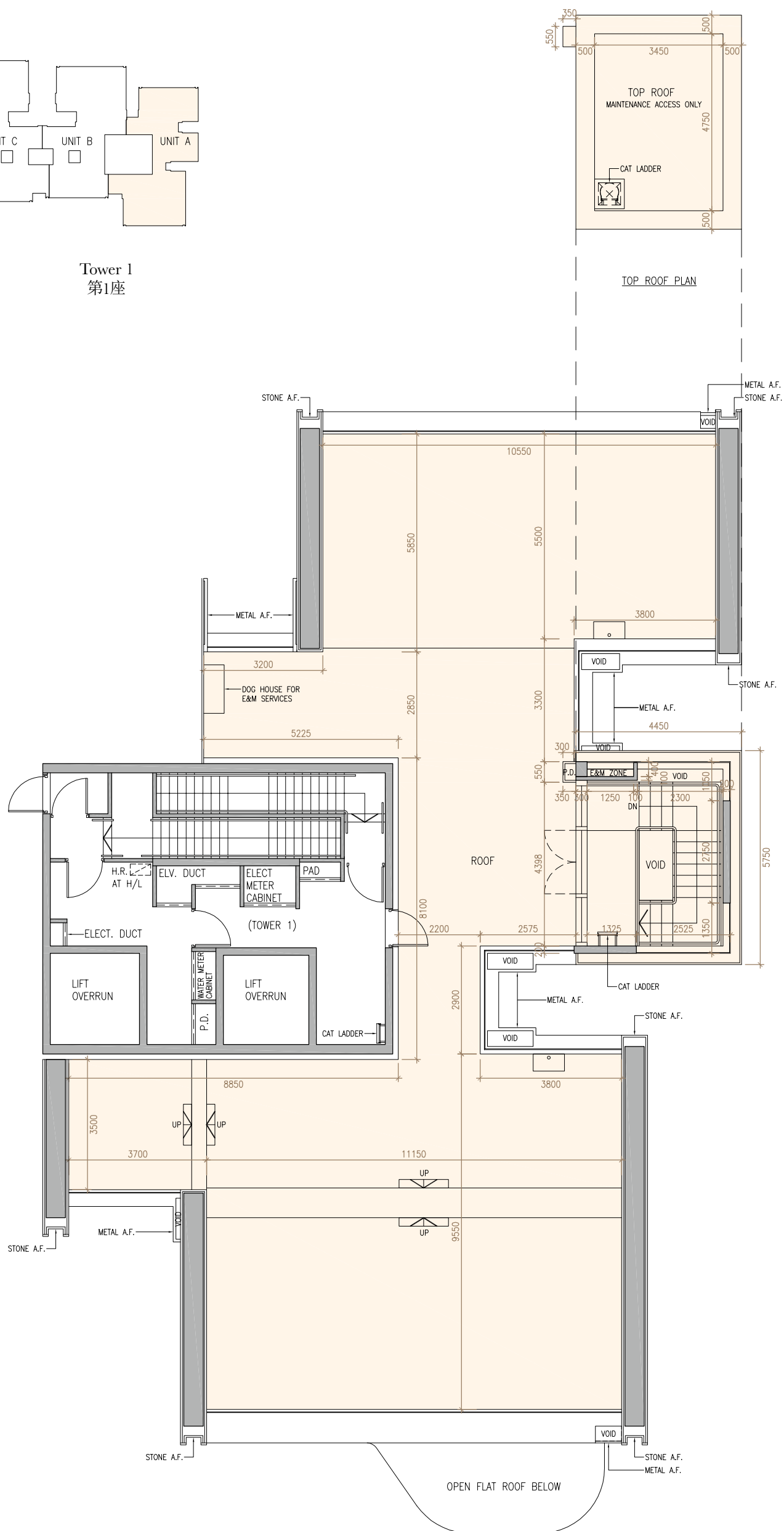
PENTHOUSE A ROOF FLOOR PLAN 頂層單位 A 天台樓面平面圖
