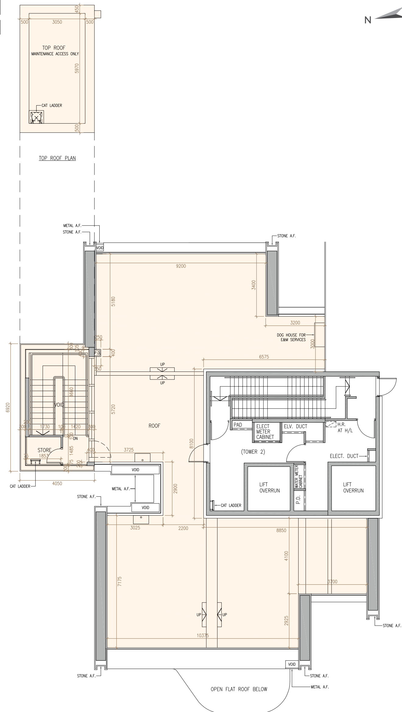
PENTHOUSE D ROOF FLOOR PLAN 頂層單位 D 天台樓面平面圖
