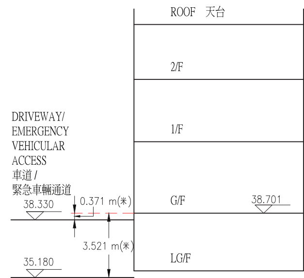
CROSS - SECTION PLAN B 橫截面圖 B
