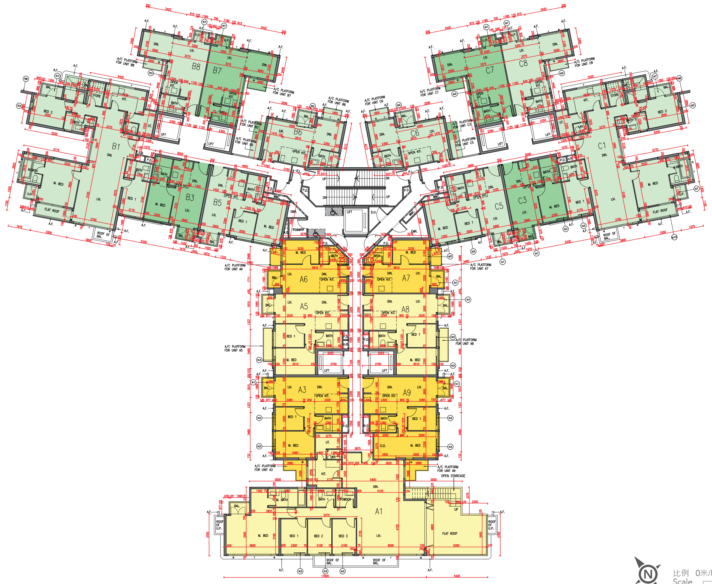
第2座17樓平面圖 Tower 2, 17/F Floor Plan
