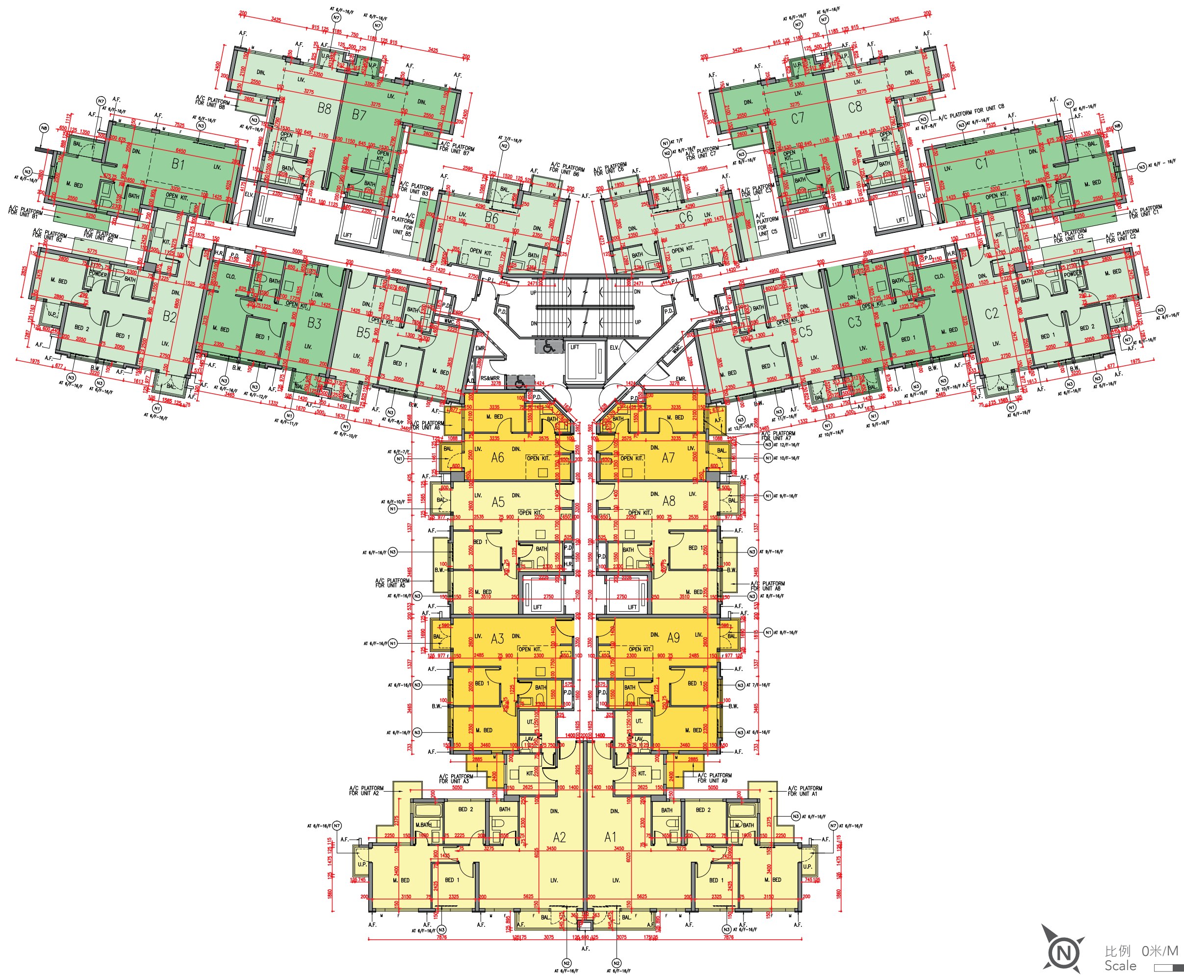
第2座6樓至16樓平面圖 Tower 2, 6/F - 16/F Floor Plan
