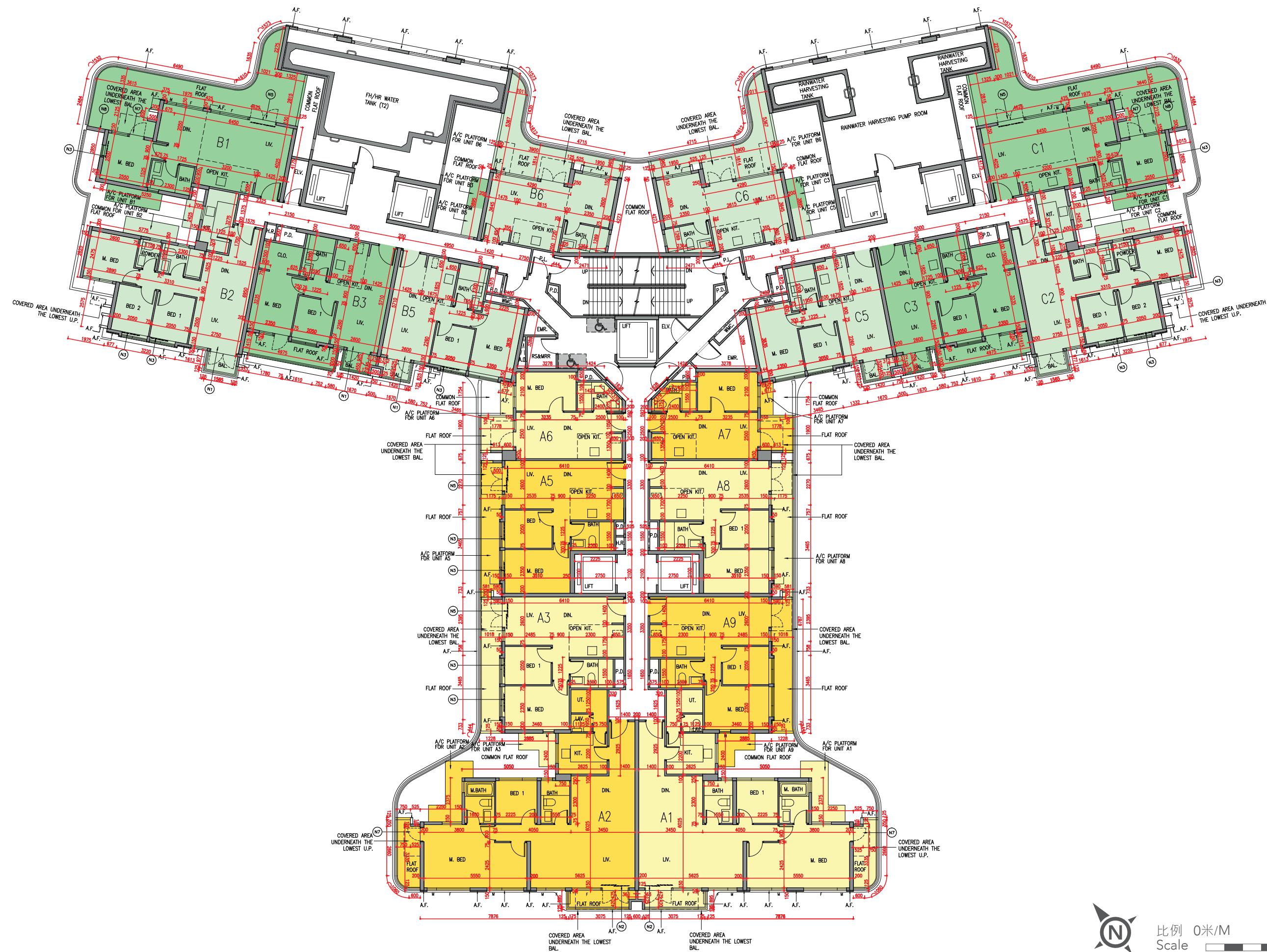
第2座5樓平面圖 Tower 2, 5/F Floor Plan
