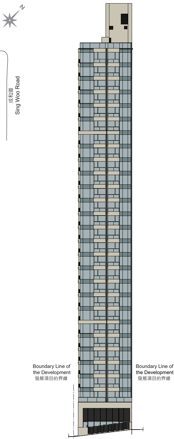
Elevation Plan D 立面圖 D
