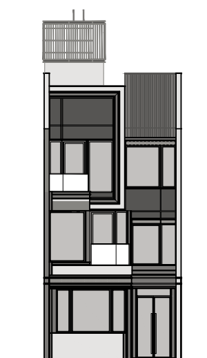
Elevation 3 立面3
