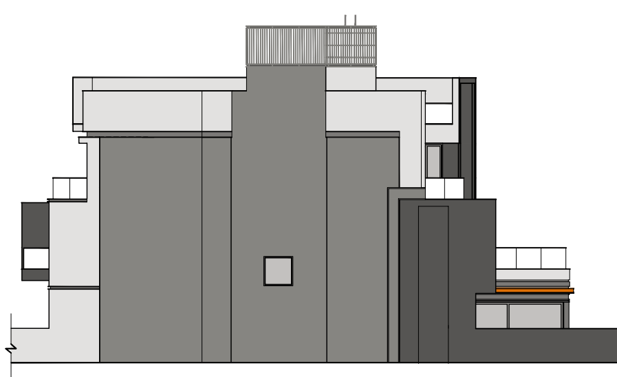
Elevation 4 立面4
