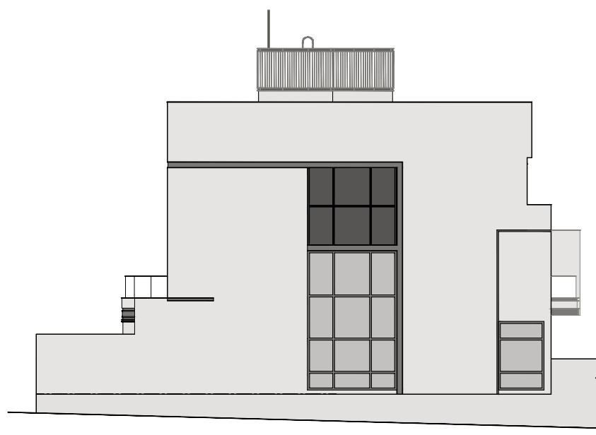
Elevation 2 立面2
