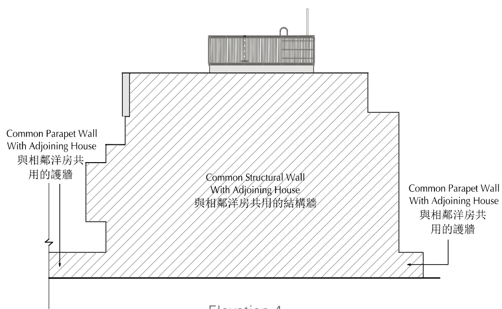
Elevation 4 立面4
