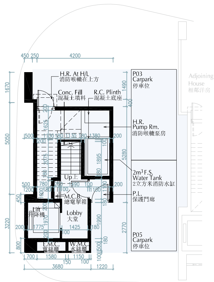
B/F Plan 地庫平面圖
