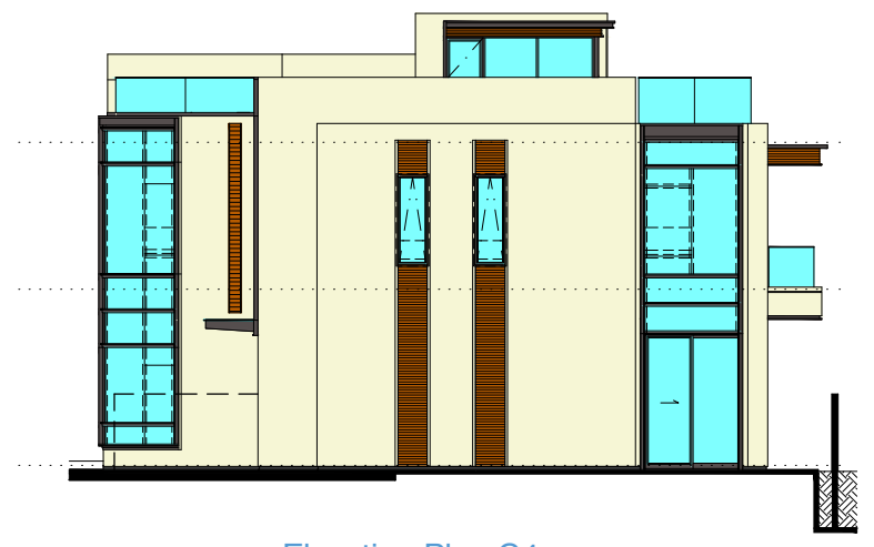
Elevation Plan C4 立面圖 C4
