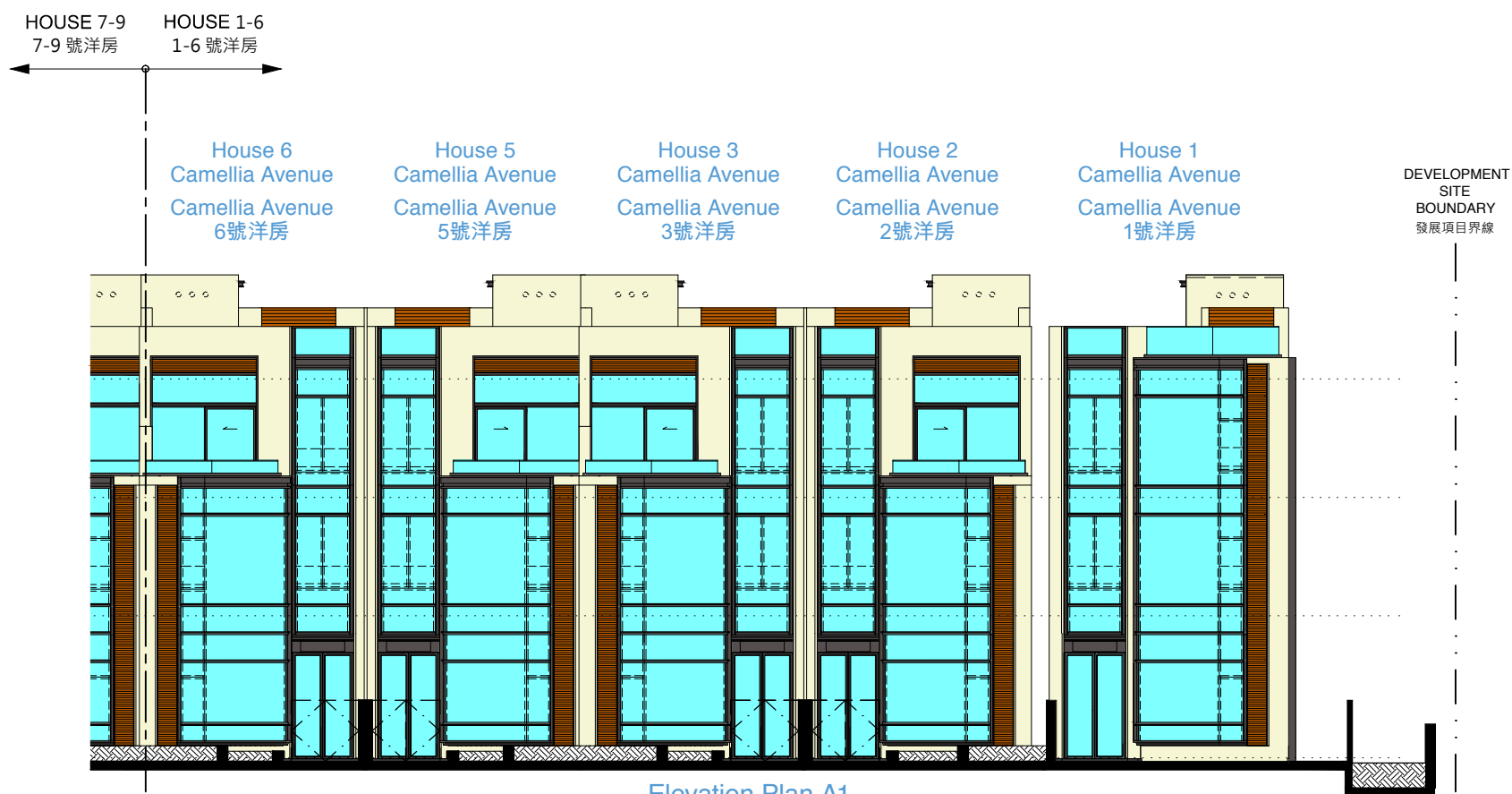
Elevation Plan A1 立面圖 A1
