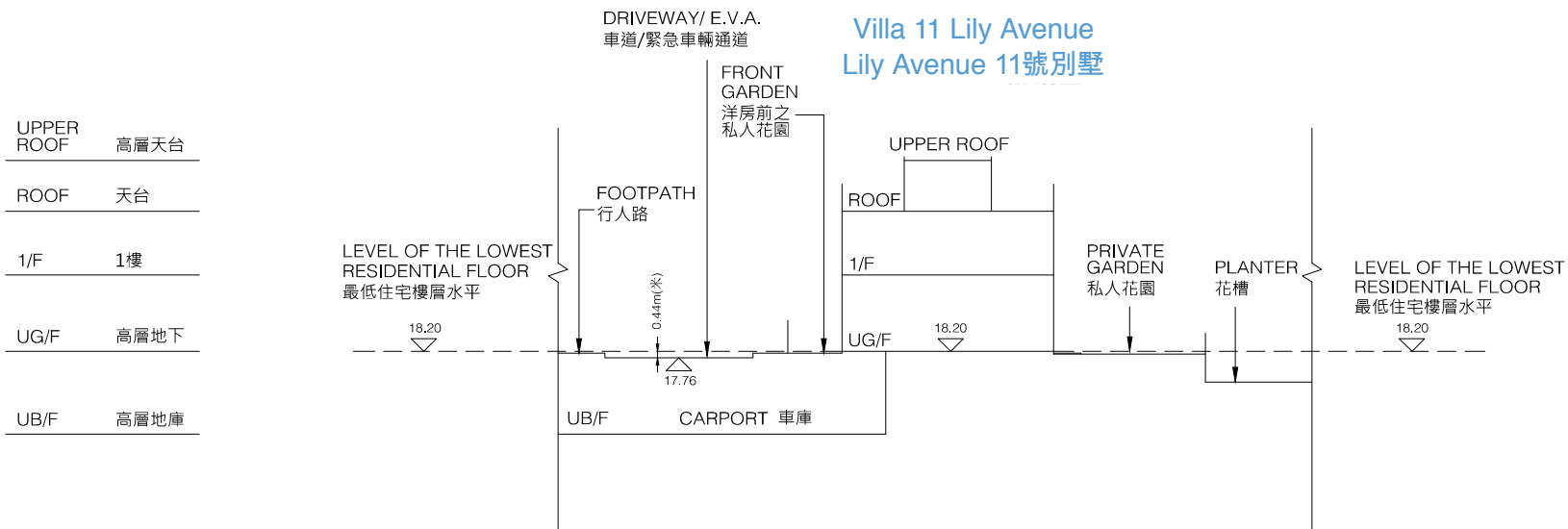
Cross - Section Plan B 橫截面圖 B
