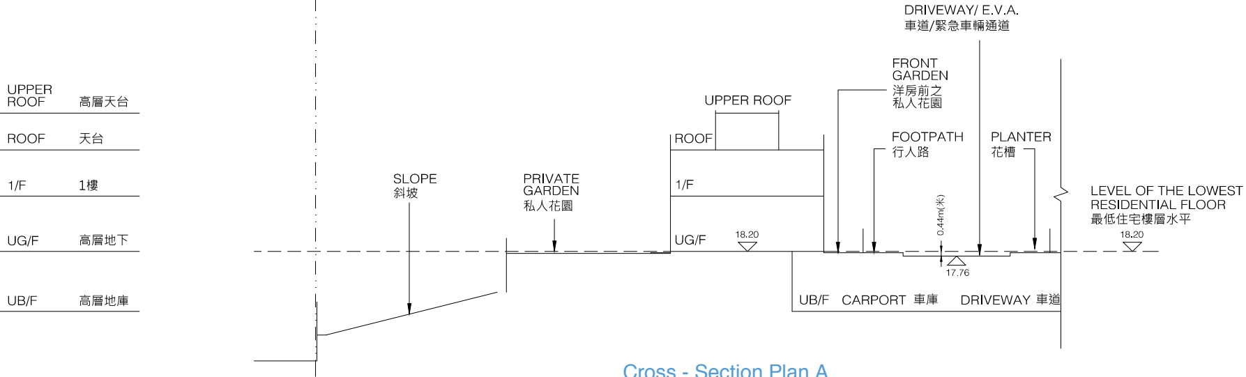
Cross - Section Plan A 橫截面圖 A
