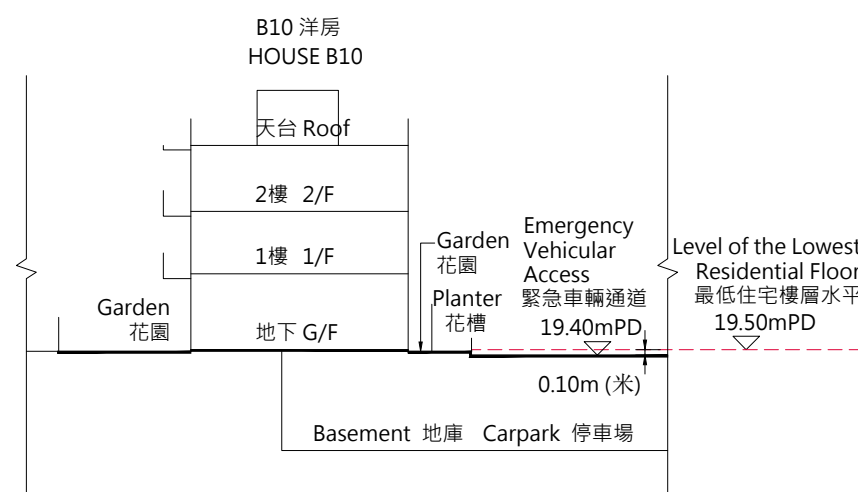
Cross-section Plan B10 橫截面圖 B10
