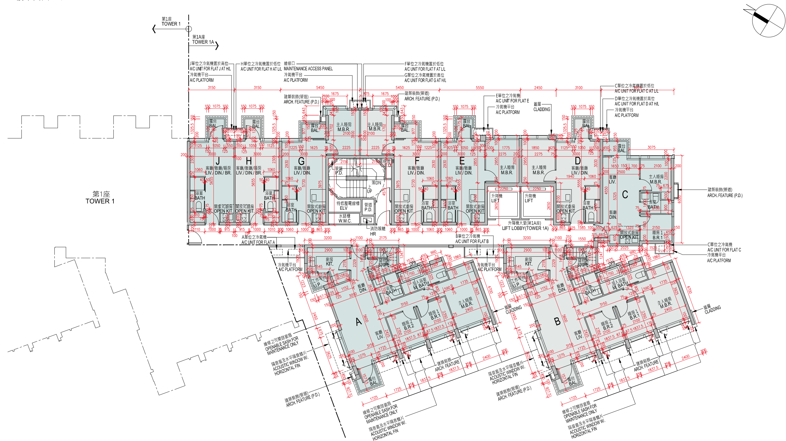
第1A座 TOWER 1A 22樓平面圖 22/F PLAN
