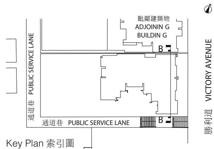
CROSS-SECTION PLAN B-B 橫截面圖 B-B
