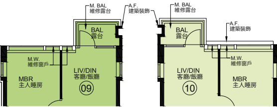
TOWER 6 5/F PART PLAN 第6座 - 5樓部份平面圖
