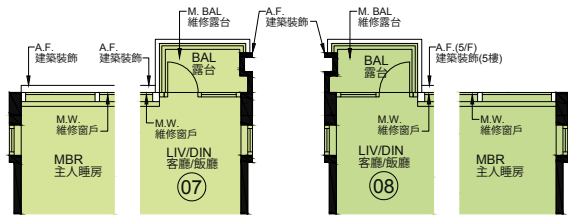
TOWER 6 3/F PART PLAN 第6座 - 3樓部份平面圖
