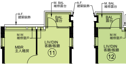
TOWER 6 3/F PART PLAN 第6座 - 3樓部份平面圖 TOWER 6 3/F, 5/F PART PLAN 第6座 - 3樓, 5樓部份平面圖 TOWER 6 3/F, 5/F PART PLAN 第6座 - 3樓, 5樓部份平面圖 TOWER 6 3/F PART PLAN 第6座 - 3樓部份平面圖 TOWER 6 5/F PART PLAN 第6座 - 5樓部份平面圖 TOWER 6 3/F, 5/F PART PLAN 第6座 - 3樓, 5樓部份平面圖 TOWER 6 3/F, 5/F PART PLAN 第6座 - 3樓, 5樓部份平面圖 TOWER 6 3/F PART PLAN 第6座 - 3樓部份平面圖 TOWER 6 3/F PART PLAN 第6座 - 3樓部份平面圖 TOWER 6 3/F, 5/F PART PLAN 第6座 - 3樓, 5樓部份平面圖 TOWER 6 3/F, 5/F PART PLAN 第6座 - 3樓, 5樓部份平面圖
