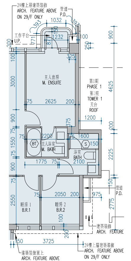
29/F Unit A Part Plan 29樓A單位之部分平面圖
