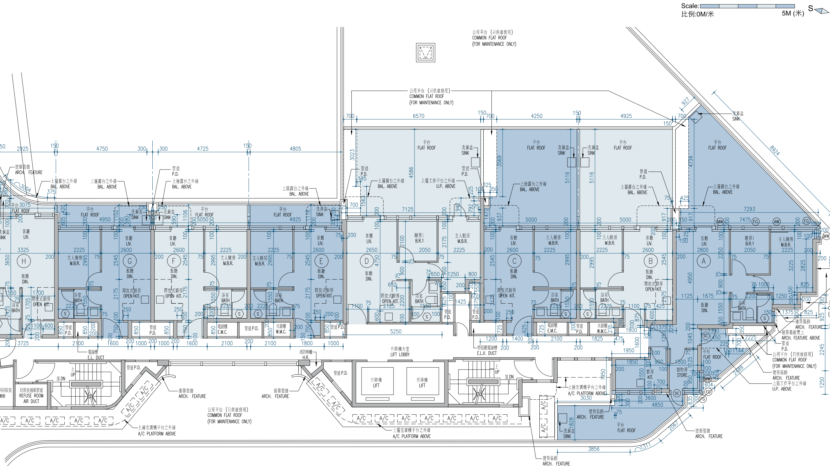
Phase 1 Tower 3(3B) 2/F Floor Plan 第1期 第3座(3B) 2樓樓面平面圖
