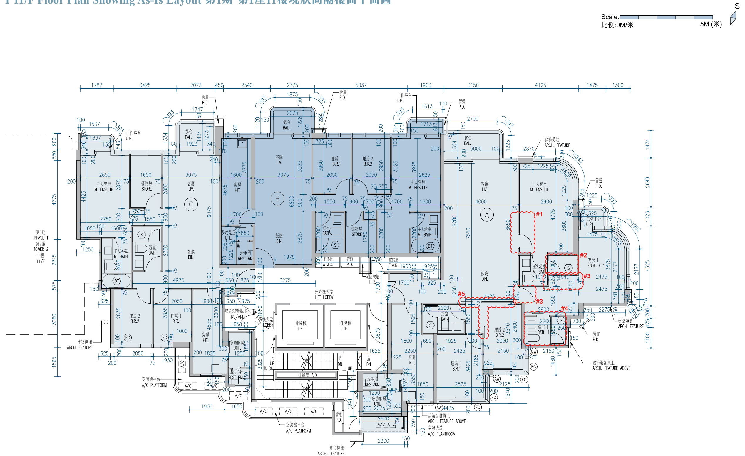
Phase 1 Tower 1 11/F Floor Plan Showing As-Is Layout 第1期 第1座11樓現狀間隔樓面平面圖
