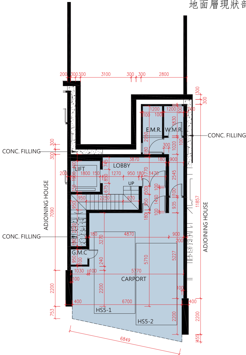
Basement Plan 地庫層平面圖
