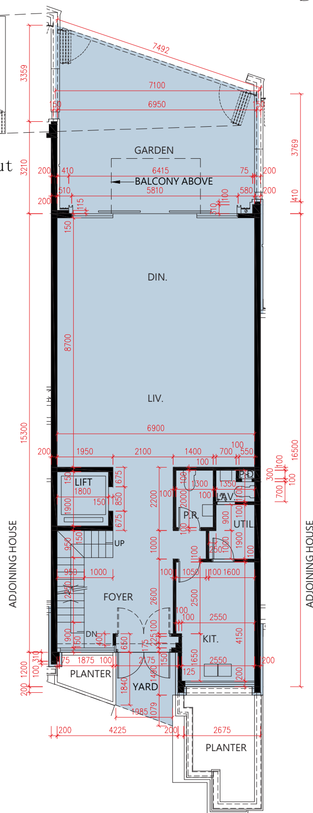
G/F Plan 地面層平面圖
