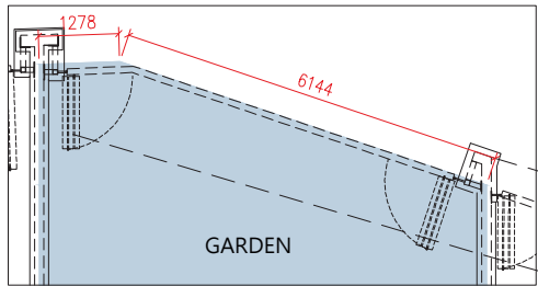
G/F Plan in "as-is" Layout 地面層現狀部分平面圖
