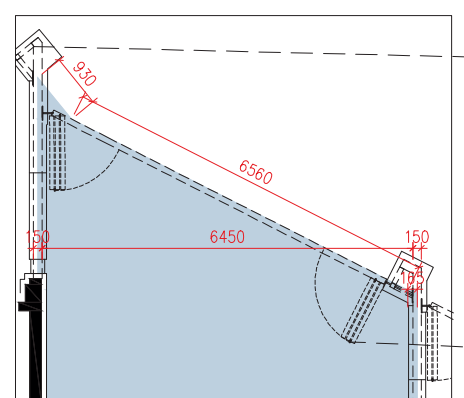
G/F Plan in "as-is" Layout 地面層現狀部分平面圖
