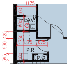
G/F Plan in "as-is" Layout 地面層現狀部分平面圖
