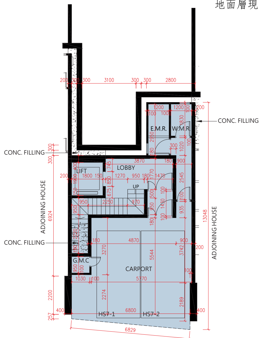
G/F Plan in "as-is" Layout 地面層現狀部分平面圖
