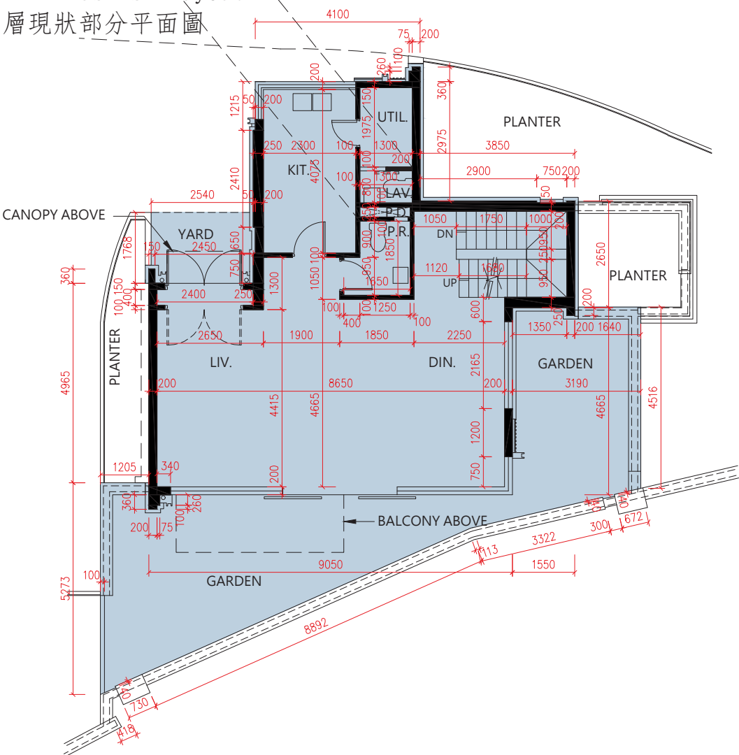
G/F Plan 地面層平面圖
