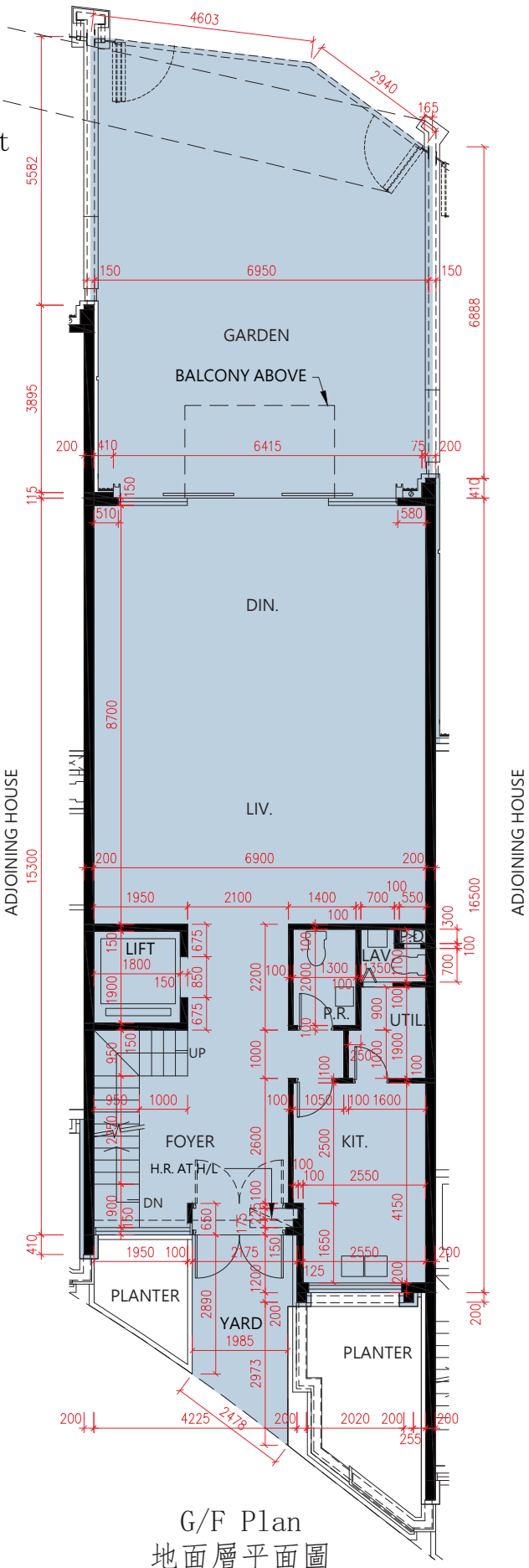
G/F Plan in "as-is" Layout 地面層現狀部分平面圖
