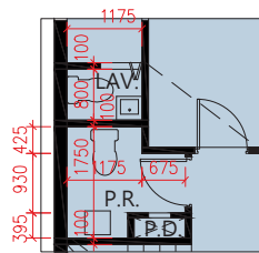
G/F Plan in "as-is" Layout 地面層現狀部分平面圖
