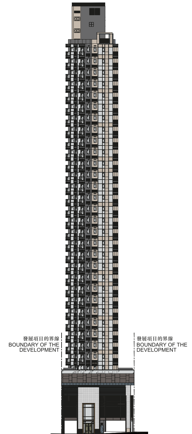
北面立面圖 NORTH ELEVATION
