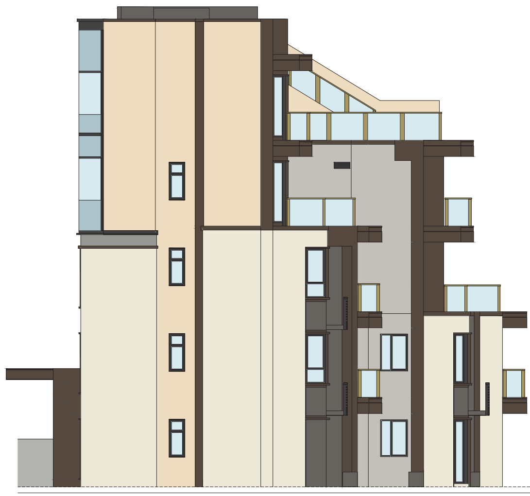
Elevation Plan P3 立面圖 P3
