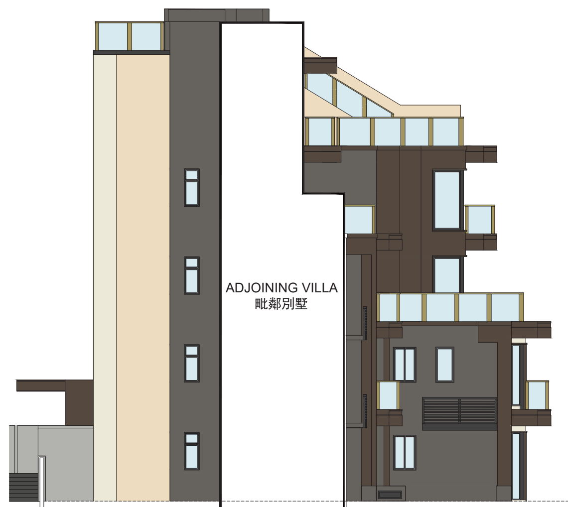
Elevation Plan K3 立面圖 K3
