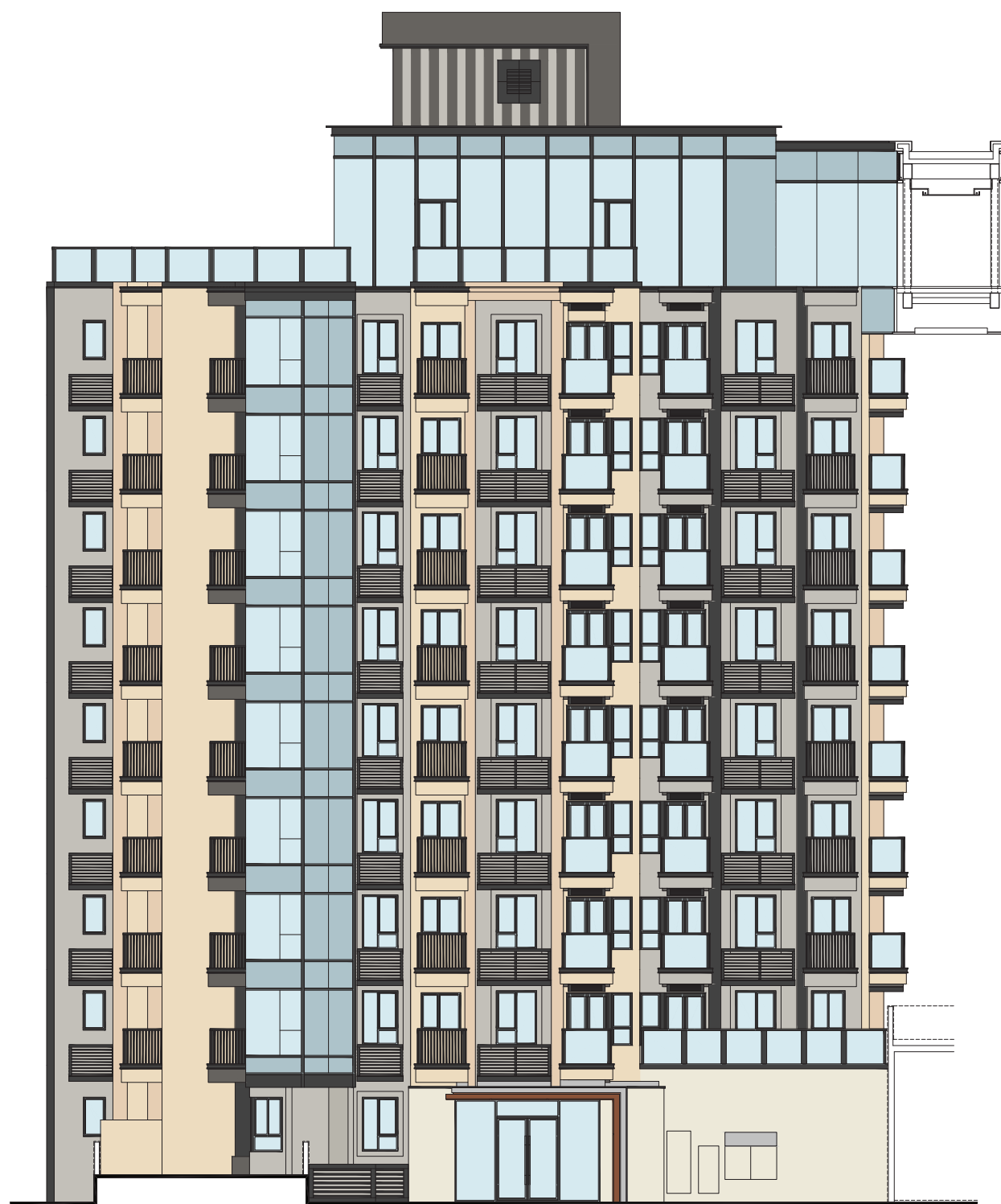
Elevation Plan F3 立面圖 F3
