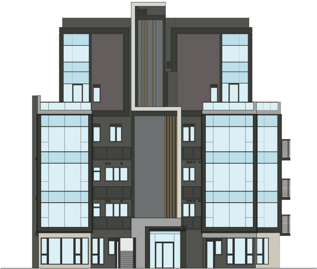
ELEVATION PLAN R1 立面圖 R1
