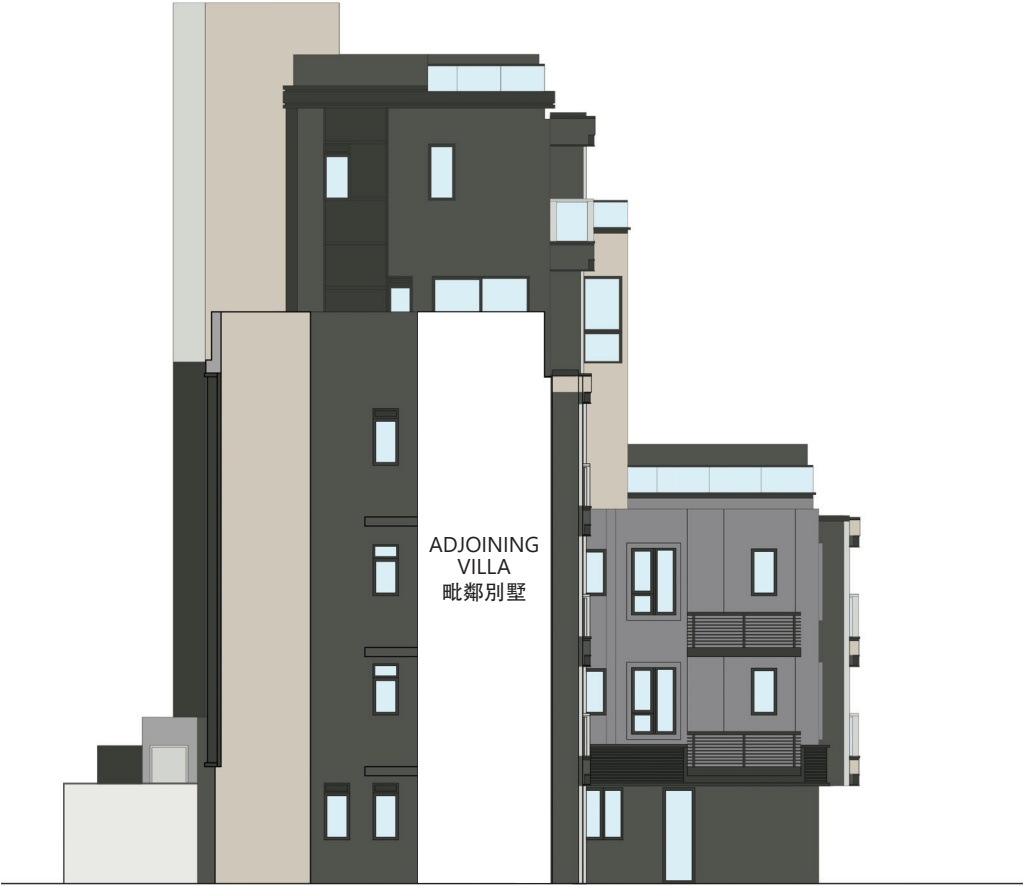
WV1 別墅WV1
