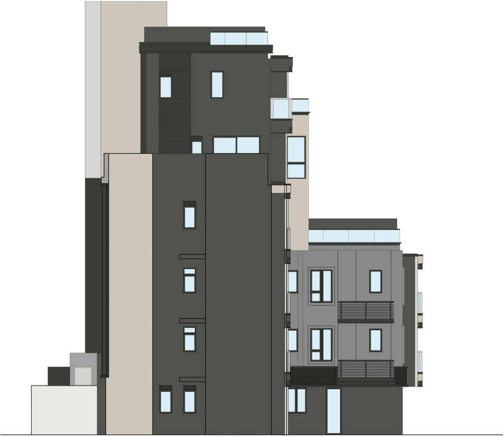
ELEVATION PLAN L2 立面圖 L2
