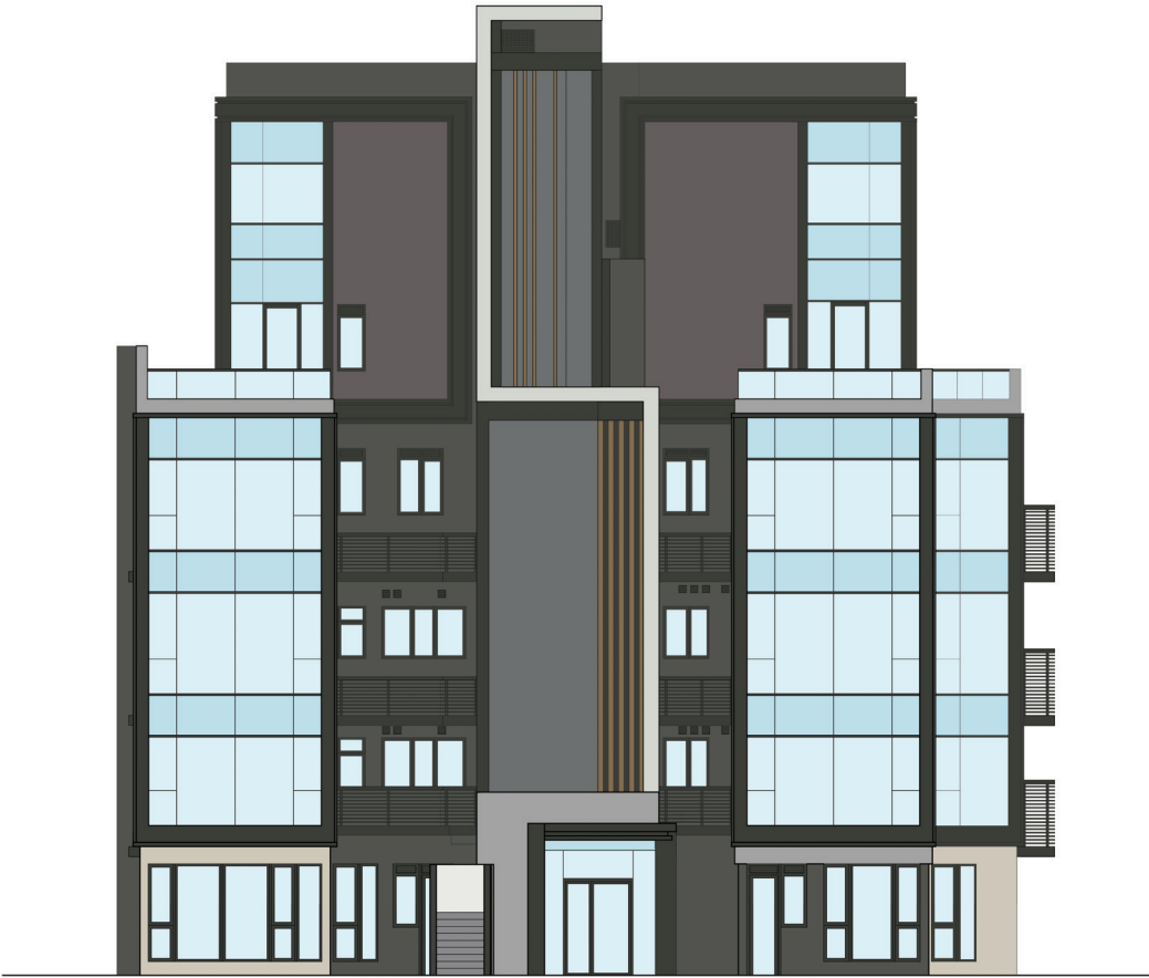
ELEVATION PLAN H1 立面圖 H1
