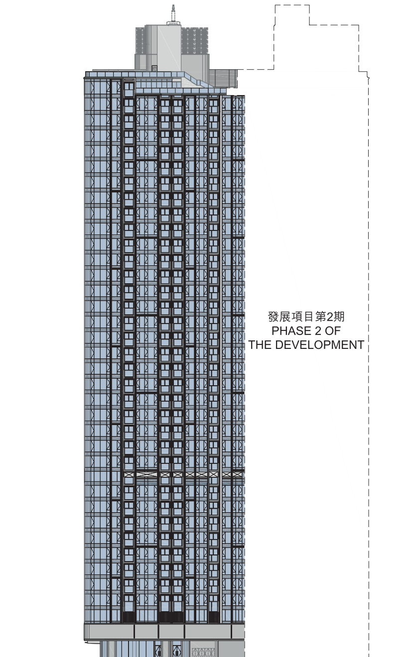
立面圖 A ELEVATION PLAN A
