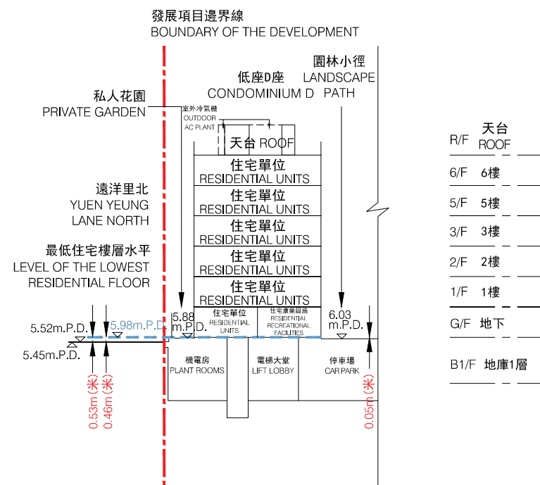
橫截面圖 G-G' Section G-G'
