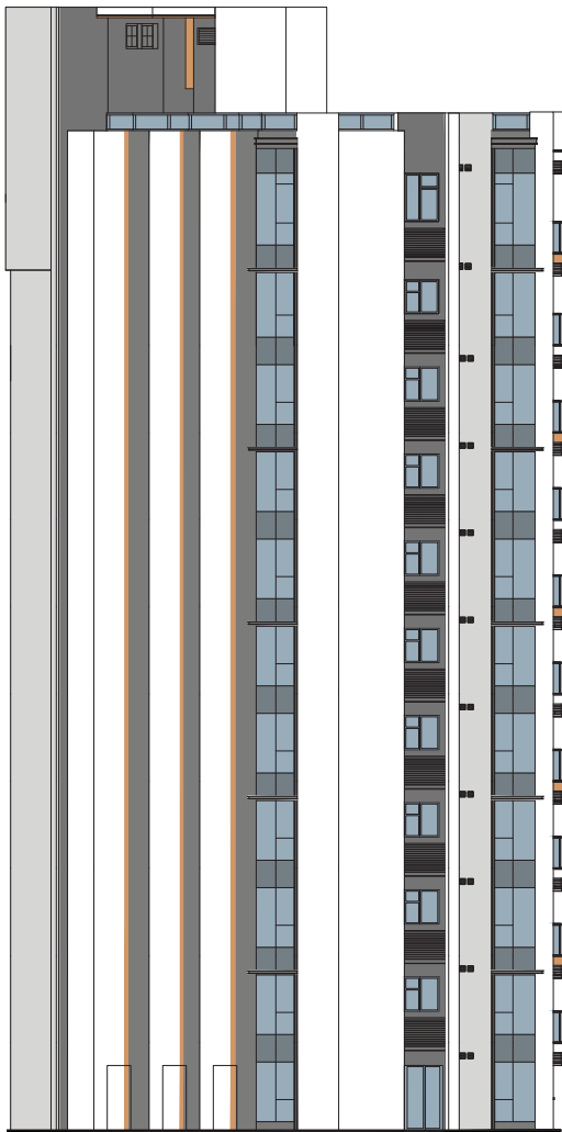
ELEVATION 6 立面 6
