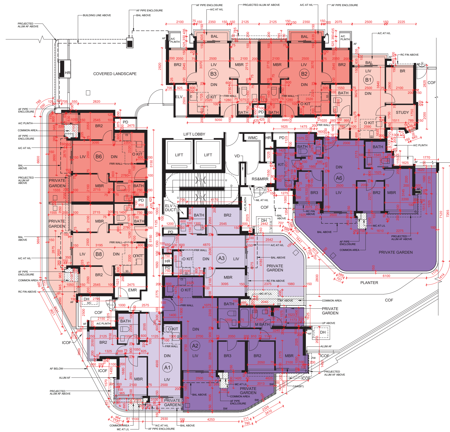
GREENWOOD TOWER 5 1/F FLOOR PLAN 翠景閣第5座 1樓平面圖
