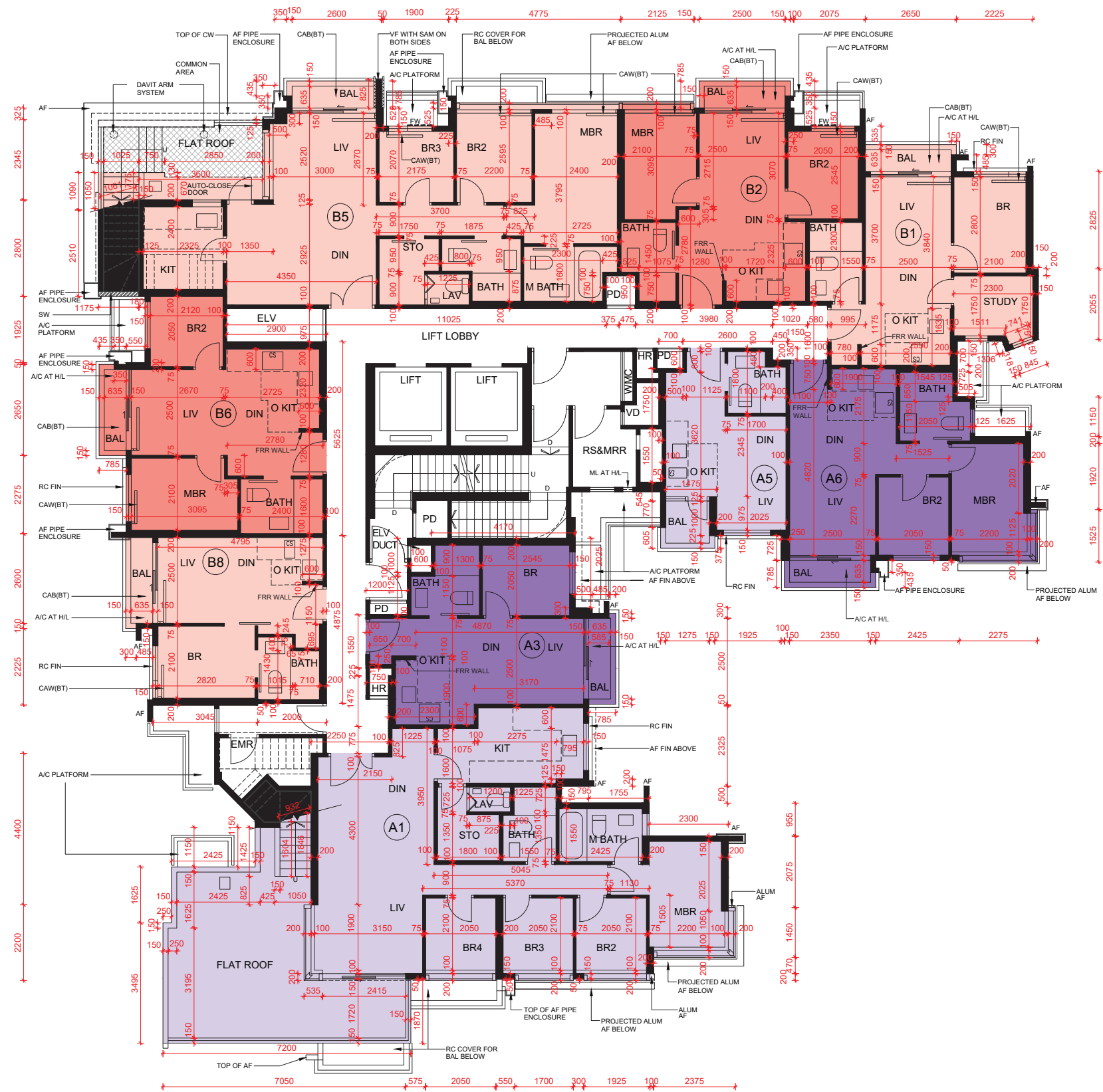
GREENWOOD TOWER 2 12/F FLOOR PLAN 翠景閣第2座 12樓平面圖
