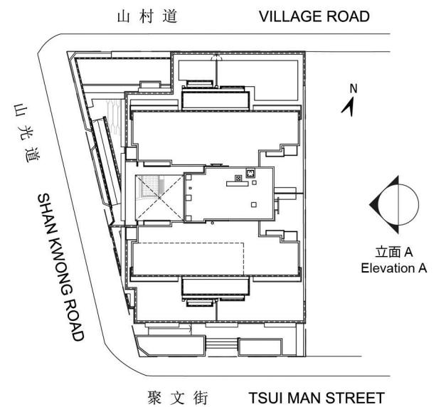
座向圖 BLOCK PLAN
