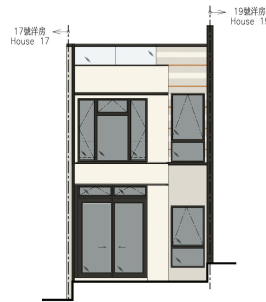
18號洋房立面圖 1 HOUSE 18 ELEVATION 1
