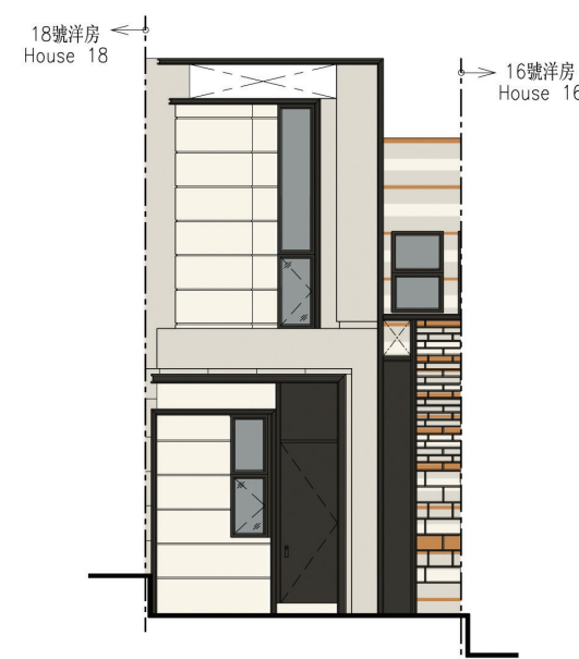
17號洋房立面圖 2 HOUSE 17 ELEVATION 2
