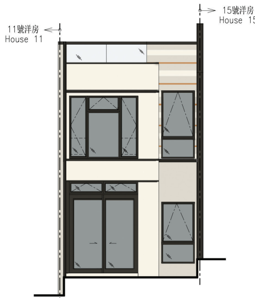
12號洋房立面圖 1 HOUSE 12 ELEVATION 1
