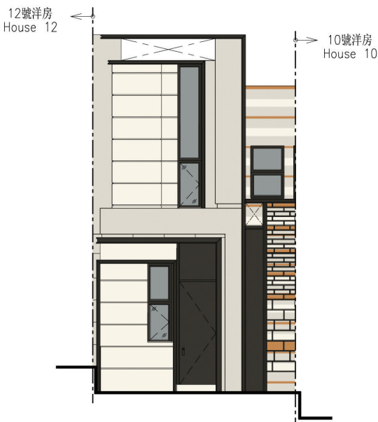
11號洋房立面圖 2 HOUSE 11 ELEVATION 2
