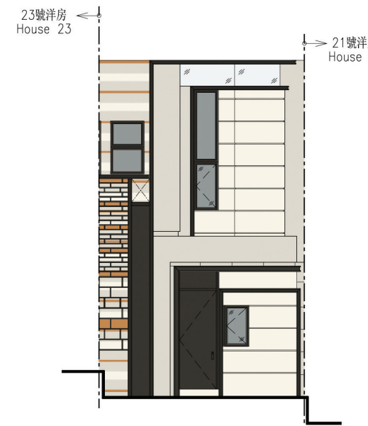
22號洋房立面圖 2 HOUSE 22 ELEVATION 2
