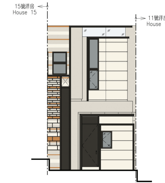
12號洋房立面圖 2 HOUSE 12 ELEVATION 2
