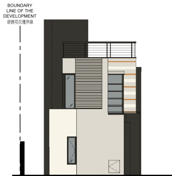
1號洋房立面圖 1 HOUSE 1 ELEVATION 1
