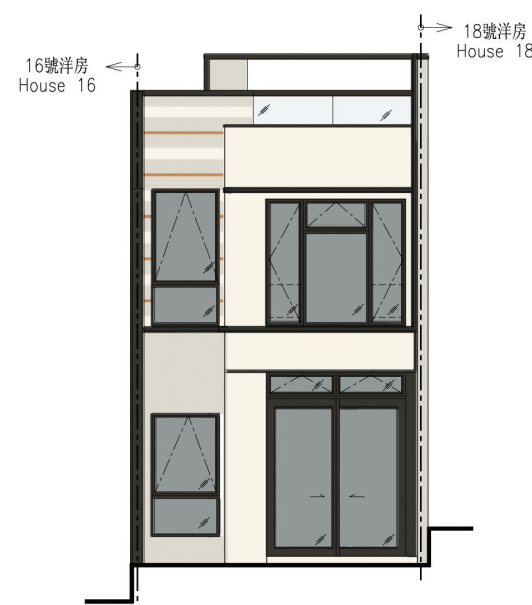
17號洋房立面圖 1 HOUSE 17 ELEVATION 1
