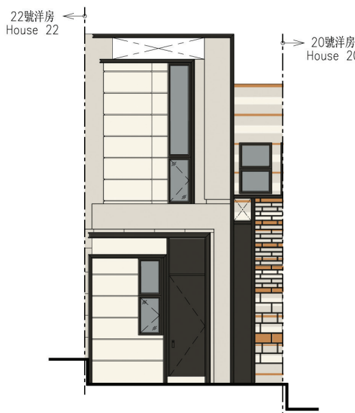
21號洋房立面圖 2 HOUSE 21 ELEVATION 2
