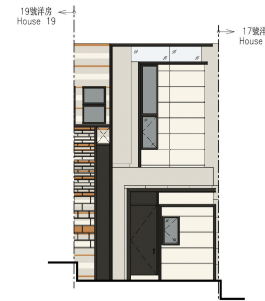
18號洋房立面圖 2 HOUSE 18 ELEVATION 2
