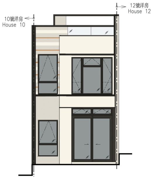
11號洋房立面圖 1 HOUSE 11 ELEVATION 1
