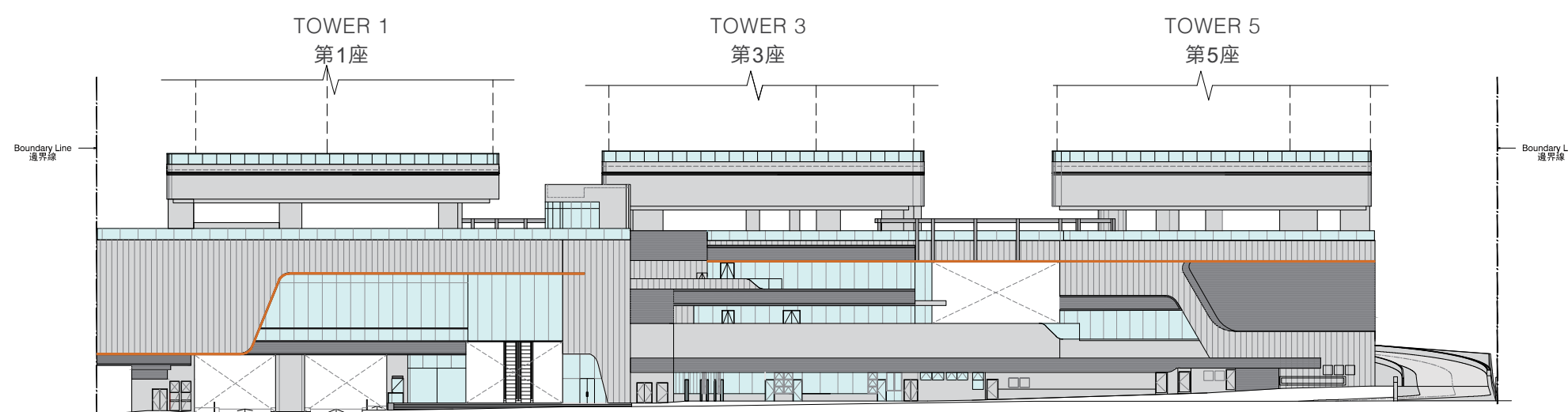
ELEVATION PLAN 2 立面圖 2
