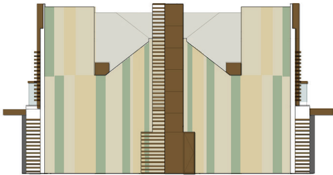
複式B座西立面圖 MAISONNETTE BUILDING B WEST ELEVATION
