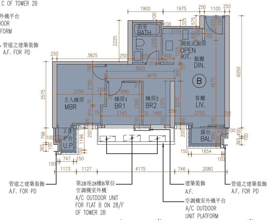
FLOOR PLAN OF FLAT B ON 28/F OF TOWER 2B 第2B座 28樓 B單位之樓面平面圖
