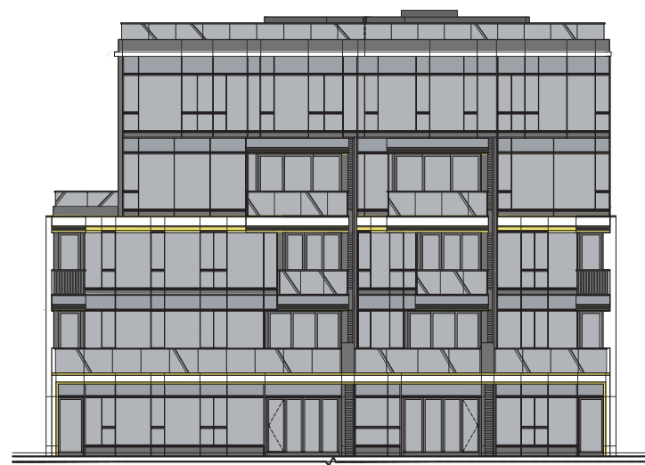
Elevation 1 立面圖1
